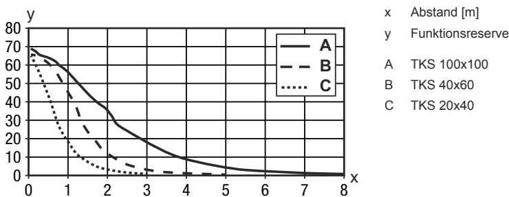
Typ. Funktionsreserve
