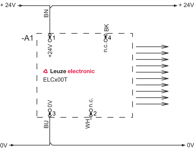
Esquema de conexión del emisor
