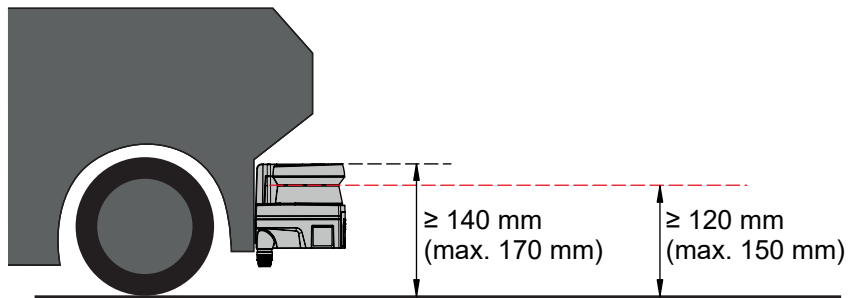
그림 6.11: 무인 수송 시스템(안전 기능 활용)을 위한 RSL 210, RSL 220 및 RSL 230의 권장 설치 높이(안전 기능 활용)
