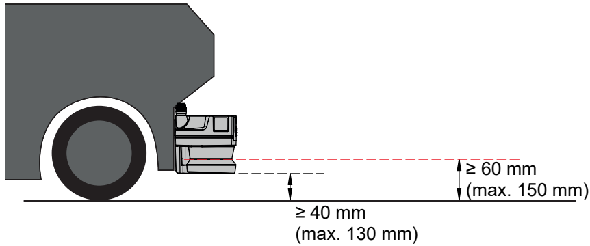
그림 6.11: 무인 수송 시스템(안전 기능 활용)을 위한 RSL 210, RSL 220 및 RSL 230의 권장 설치 높이(안전 기능 활용)
