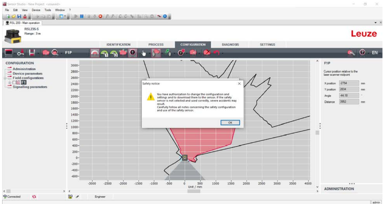
그림 8.41: 안전 구성을 다운로드하기 전 점검
