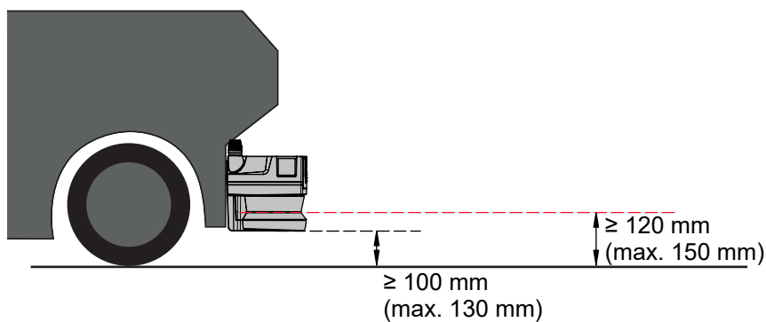
그림 6.12: 무인 수송 시스템용 RSL 235의 권장 설치 높이(안전 기능 사용 및 내비게이션 지원을 위한 측정 데이터 출력)
