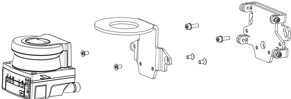
Figura 6.17: Montaggio con supporto a parete e staffa di protezione
