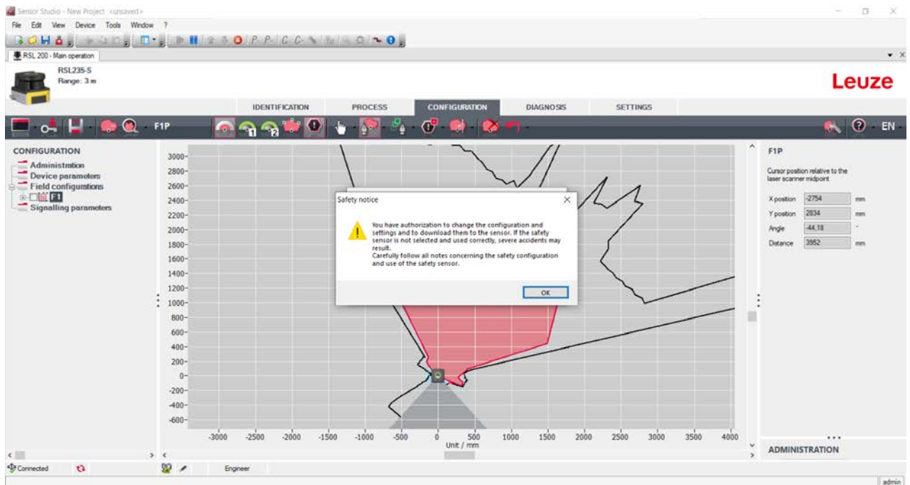
Figura 8.37: Controllo prima del download della configurazione di sicurezza
