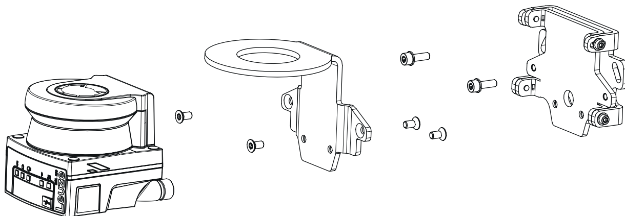
Figura 6.16: Montaggio con supporto a parete e staffa di protezione
