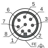
Figura 7.2: Assegnazione dei pin del connettore maschio M12, 8 poli
