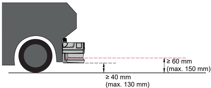
Figura 6.11: Altezza di montaggio consigliata per RSL 210, RSL 220 e RSL 230 per sistemi di trasporto senza conducente (utilizzo della funzione di sicurezza)
