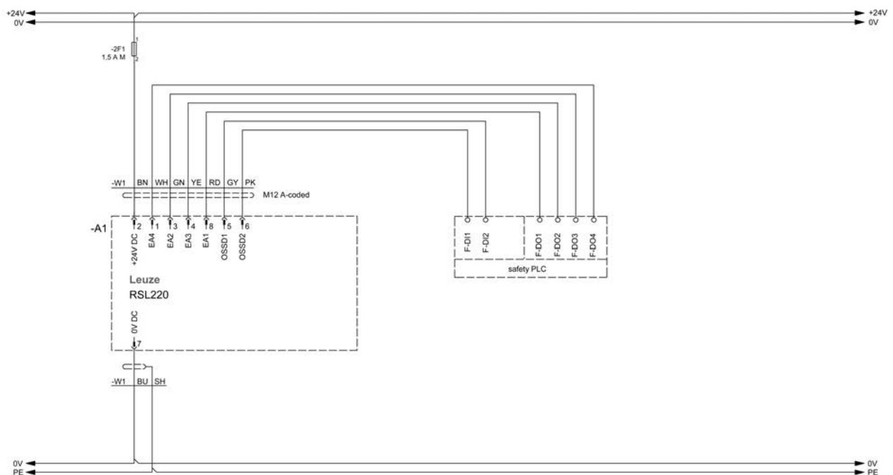
Figura 7.3: RSL 220 con sistema di controllo di sicurezza
