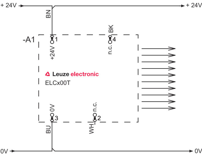
Schemat podłączania nadajnika
