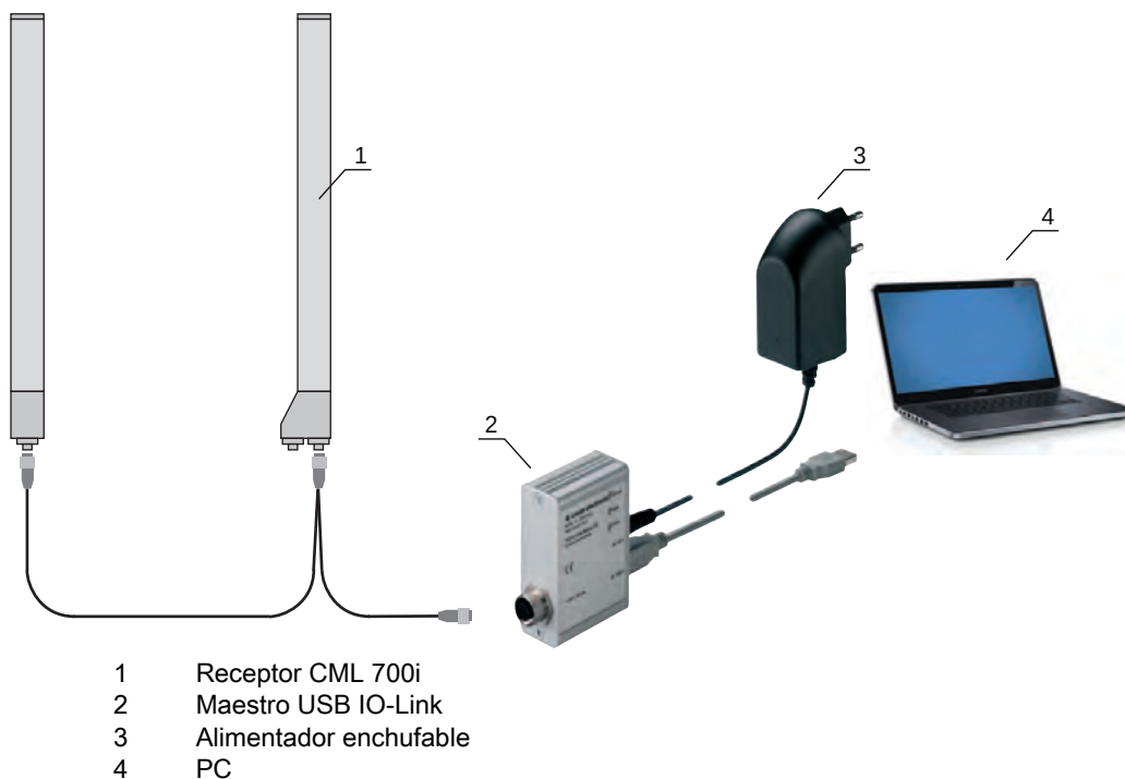
Fig. 12.2: CML 700i (bus de campo) conexión al maestro USB IO-Link
