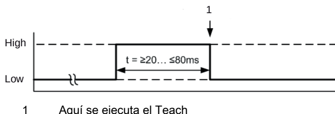
Fig. 8.6: Señales de control en Teach por cable con configuración NPN
