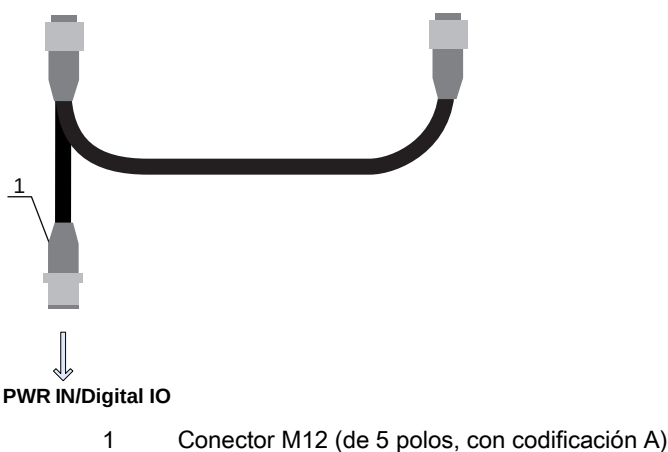
Fig. 7.7: Conexión X1 – PWR IN/Digital IO
