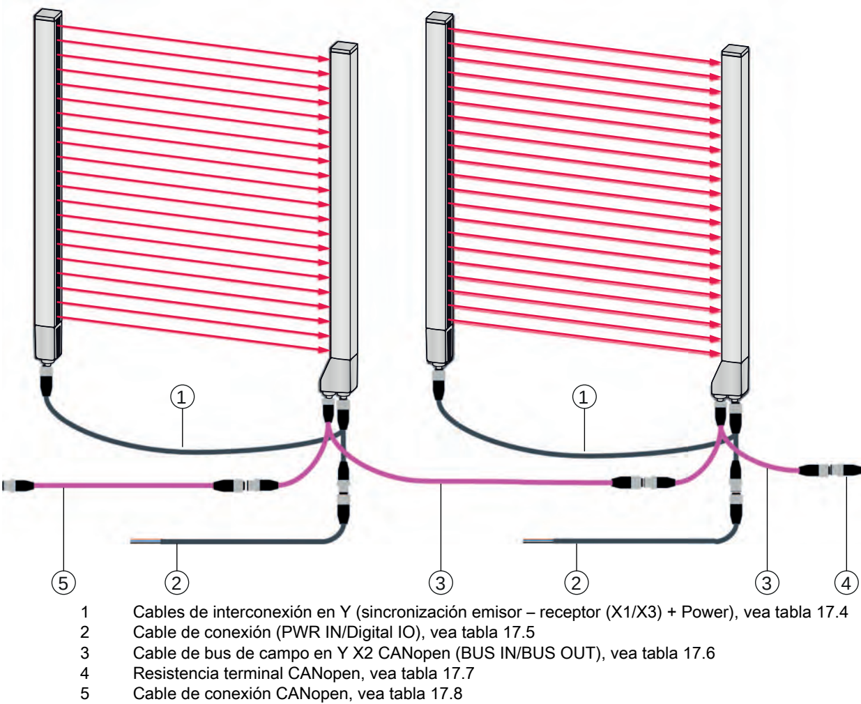
Fig. 17.1: Interfaz CANopen/IO-Link
