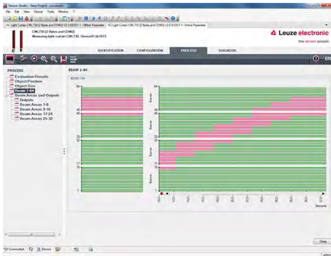
Fig. 12.7: Visualización gráfica: Representación beamstream
