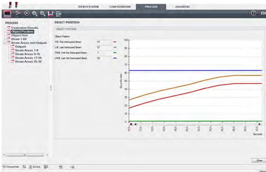
Fig. 12.6: Visualización gráfica: Posición del objeto
