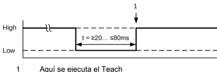
Fig. 8.5: Señales de control en Teach por cable con configuración PNP
