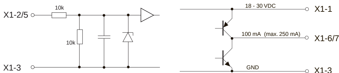
Bild 7.4: Prinzipdarstellung Digitale Ein-/Ausgänge
