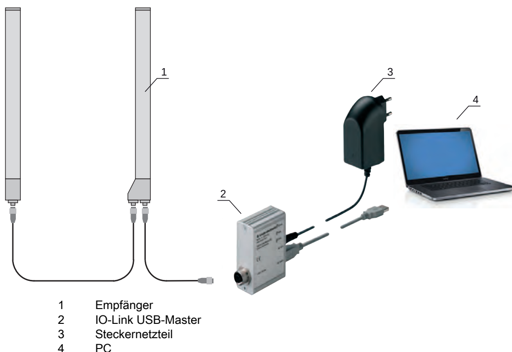
Bild 16.2: CML 700i (Analog/IO-Link) Anschluss an den IO-Link USB-Master
