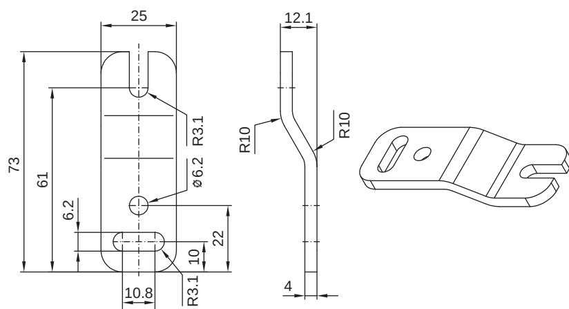
Bild 20.4: Parallelhalterung BT-2Z
