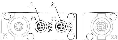
Bild 7.17: X2-Anschlüsse – CML 700i mit PROFINET-Schnittstelle
