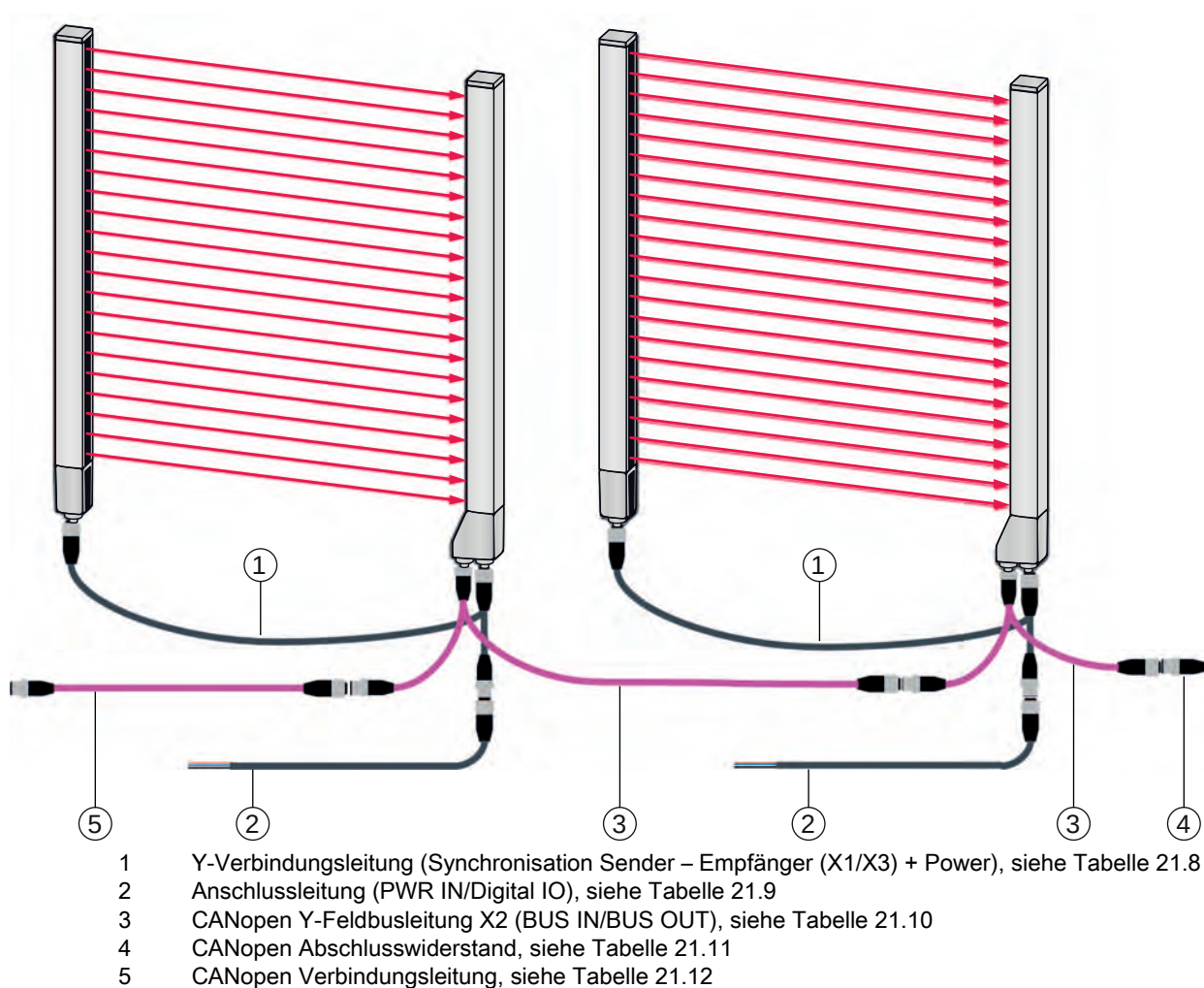
Bild 21.4: CANopen-Schnittstelle
