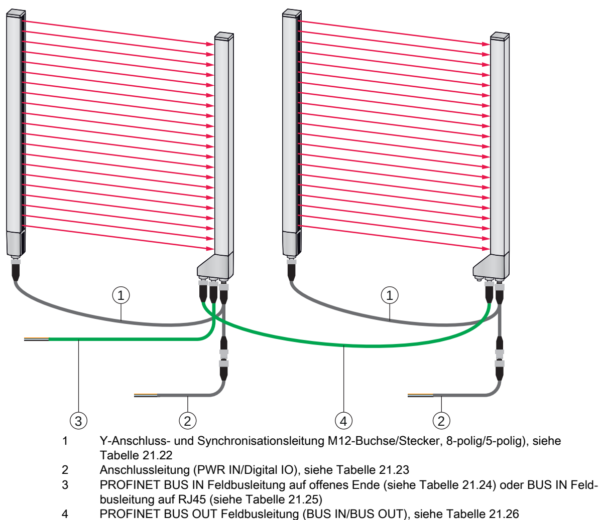
Bild 21.7: PROFINET-Schnittstelle
