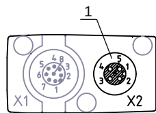
1 M12-Buchse (5-polig, A-kodiert) Bild 7.8: X2-Anschluss – CML 720i Ex mit CANopen-Schnittstelle
