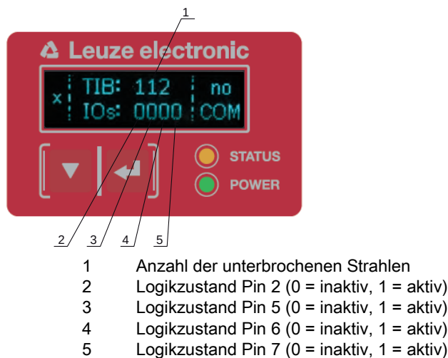
Bild 3.5: OLED-Display am Empfänger im Prozessbetrieb
