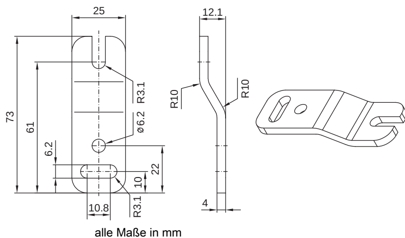
Bild 16.3: Parallelhalterung BT-2Z
