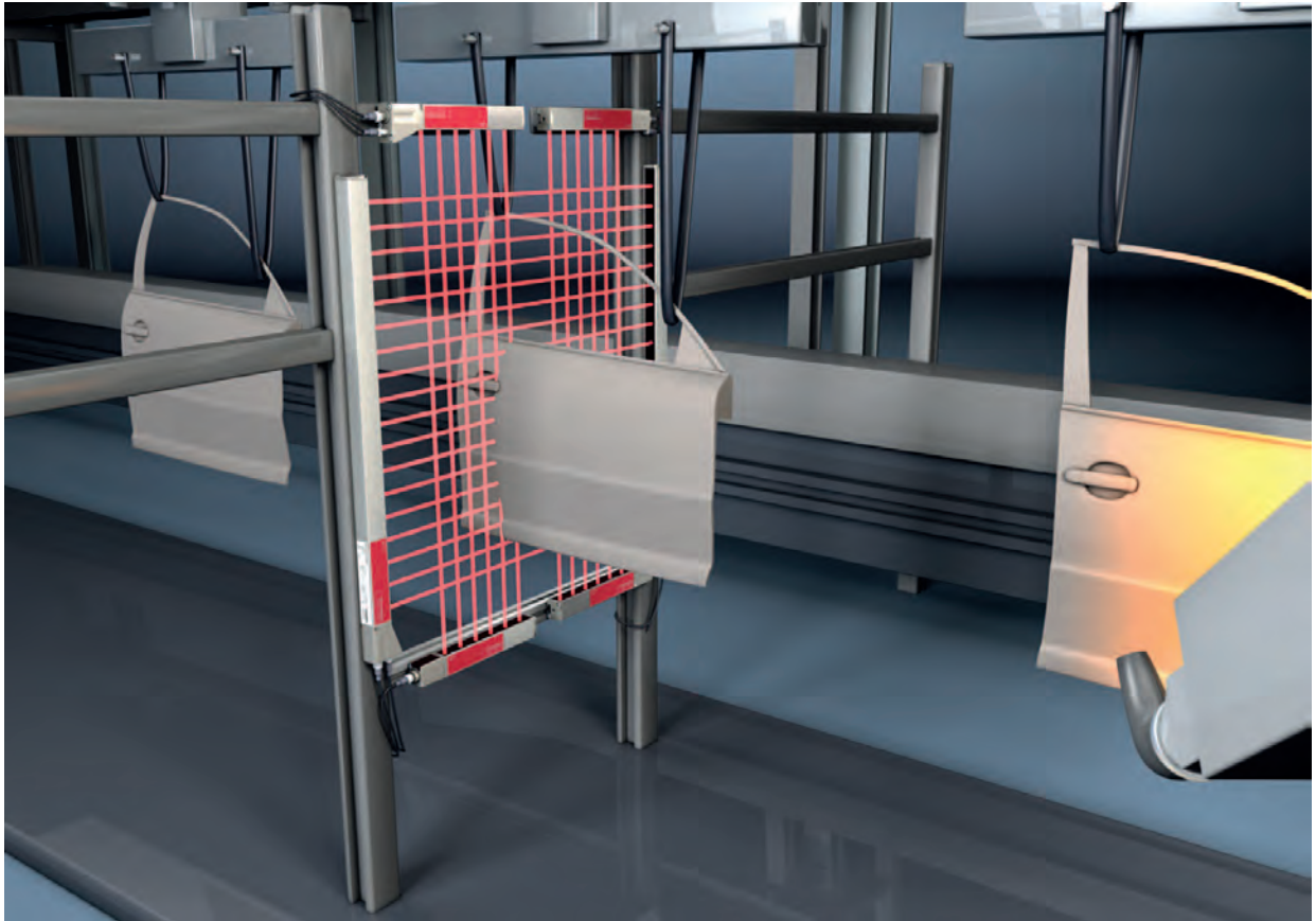
Bild 5.4: Konturvermessung
