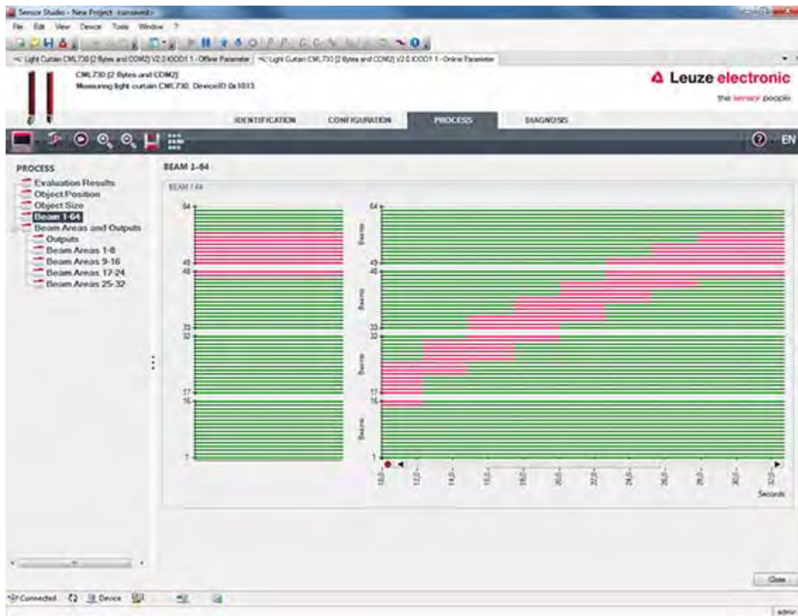
Bild 12.6: Grafische Visualisierung: Beamstream-Darstellung
