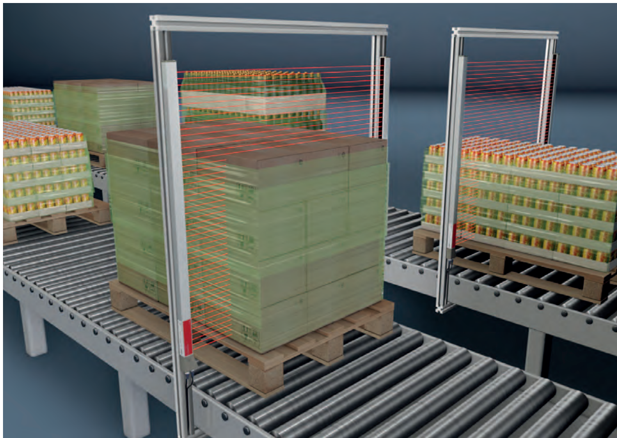
Bild 5.1: Höhenmessung
