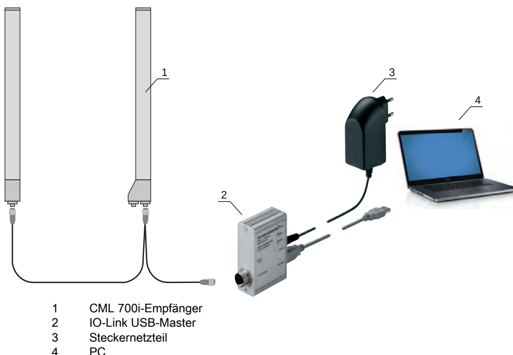
Bild 12.2: CML 700i (Feldbus) Anschluss an den IO-Link USB-Master
