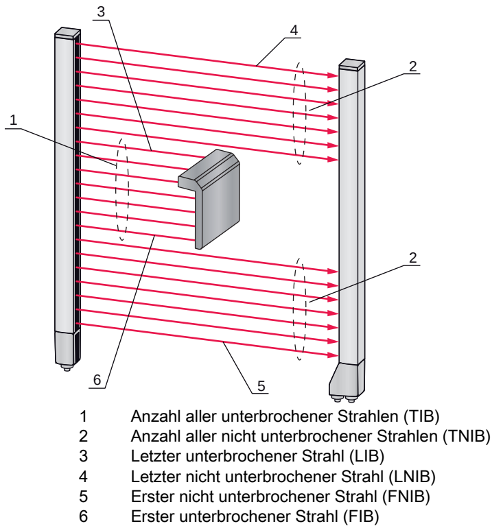
Bild 4.5: Auswertefunktionen
