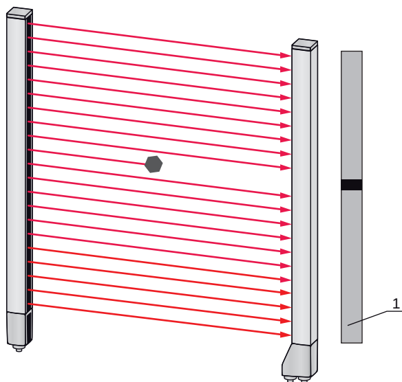
Bild 4.7: Smoothing-Konfiguration „1“
