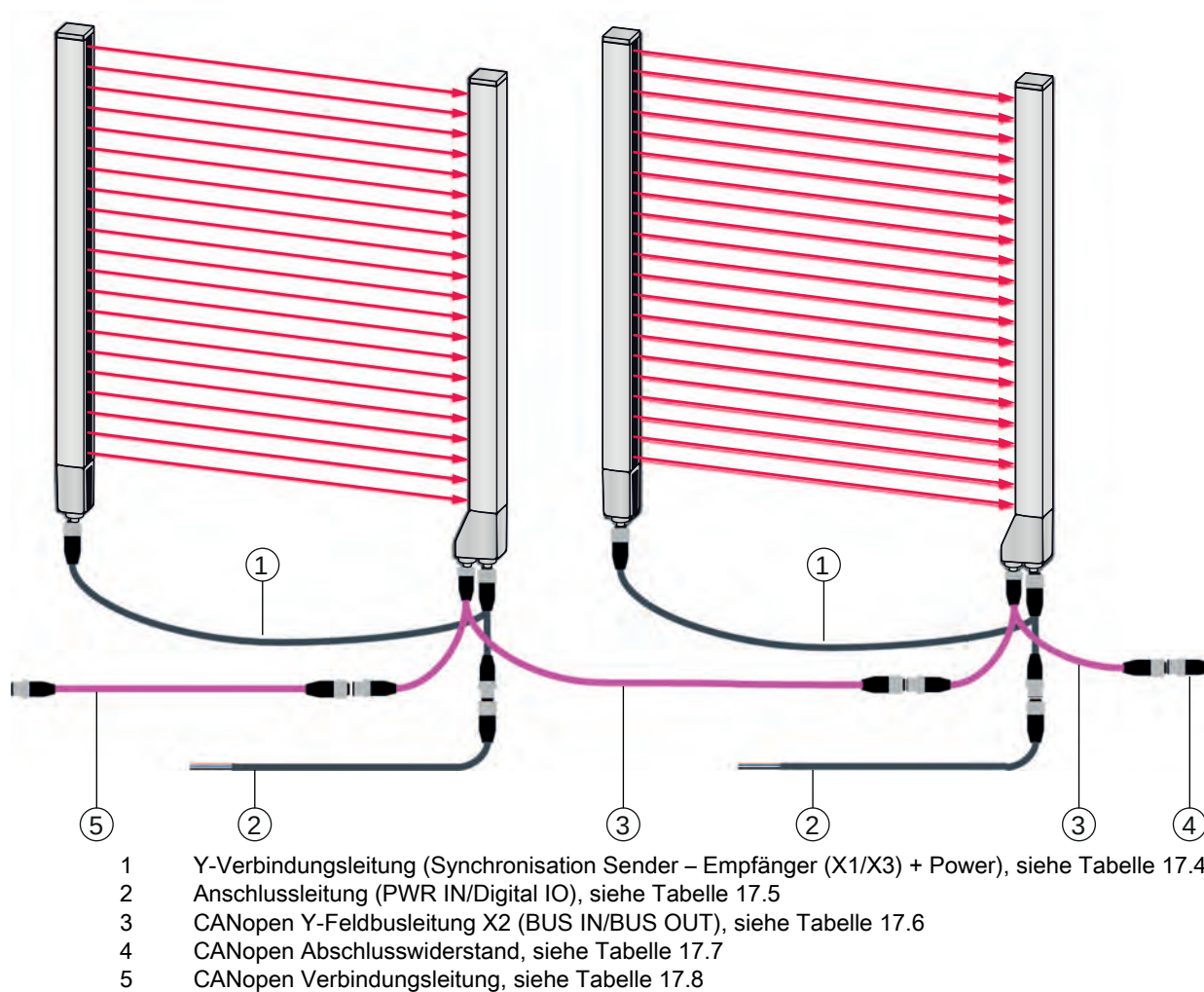
Bild 17.1: CANopen/IO-Link-Schnittstelle
