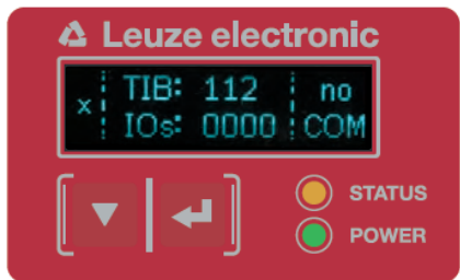
Bild 3.6: Funktionstasten am Empfänger
