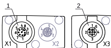
Bild 7.6: X1/X3-Anschluss
