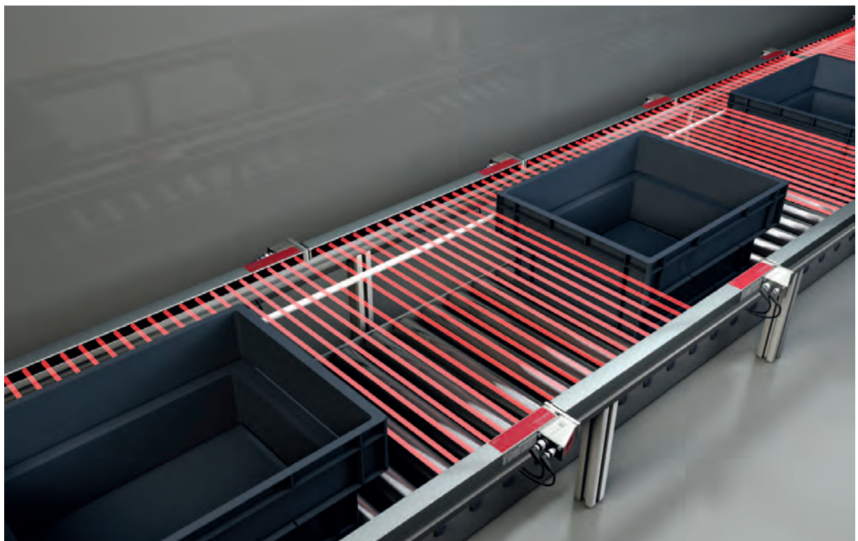
Bild 5.5: Lückensteuerung/Lückenvermessung
