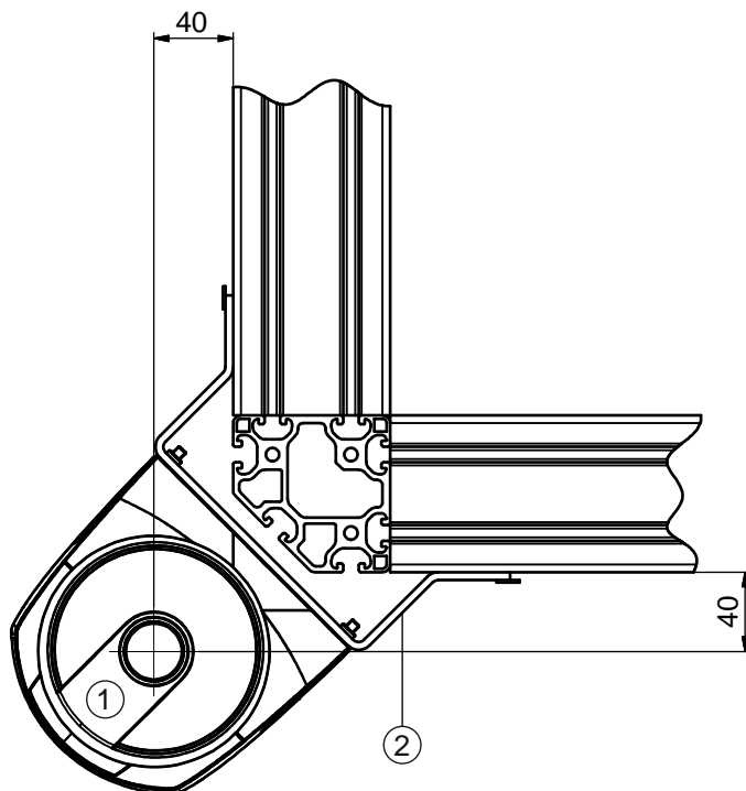
Fig. 7.3: Exemple : montage sur un montant
