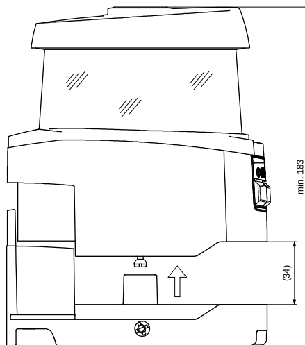
Resim 15.2: Bağlantı ünitesi emniyet lazer alan tarayıcısı montaj ölçüleri
