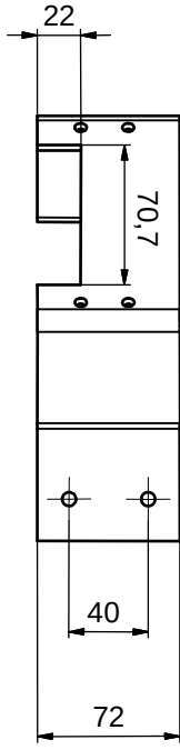
Resim 15.12: Montaj dirseği BT856M, görünüm A
