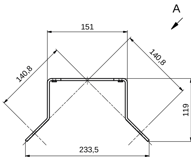
Figura 15.10: Escuadra de montaje BT840M, vista A
