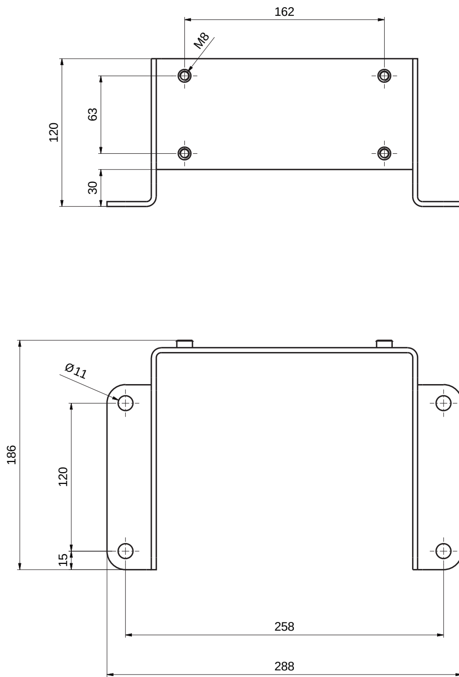
Figura 15.6: Escuadra de montaje BTF815M
