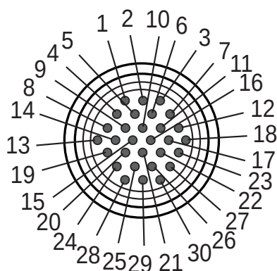
Figura 8.1: Asignación de pines de conector M30, de 30 polos
