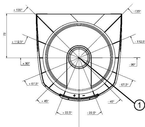
Figura 15.3: Espacio mínimo requerido para el montaje y la sustitución del escáner
