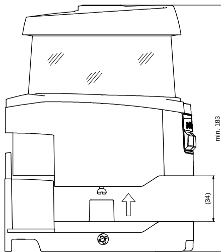
Figura 15.2: Medidas de montaje del escáner láser de seguridad con unidad de conexión
