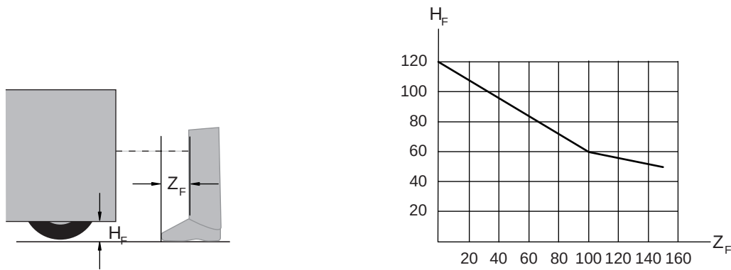
Figura 7.15: Diagrama para la determinación del suplemento Z_{\text{F}} cuando no hay suficiente altura sobre el suelo H_{\text{F}}
