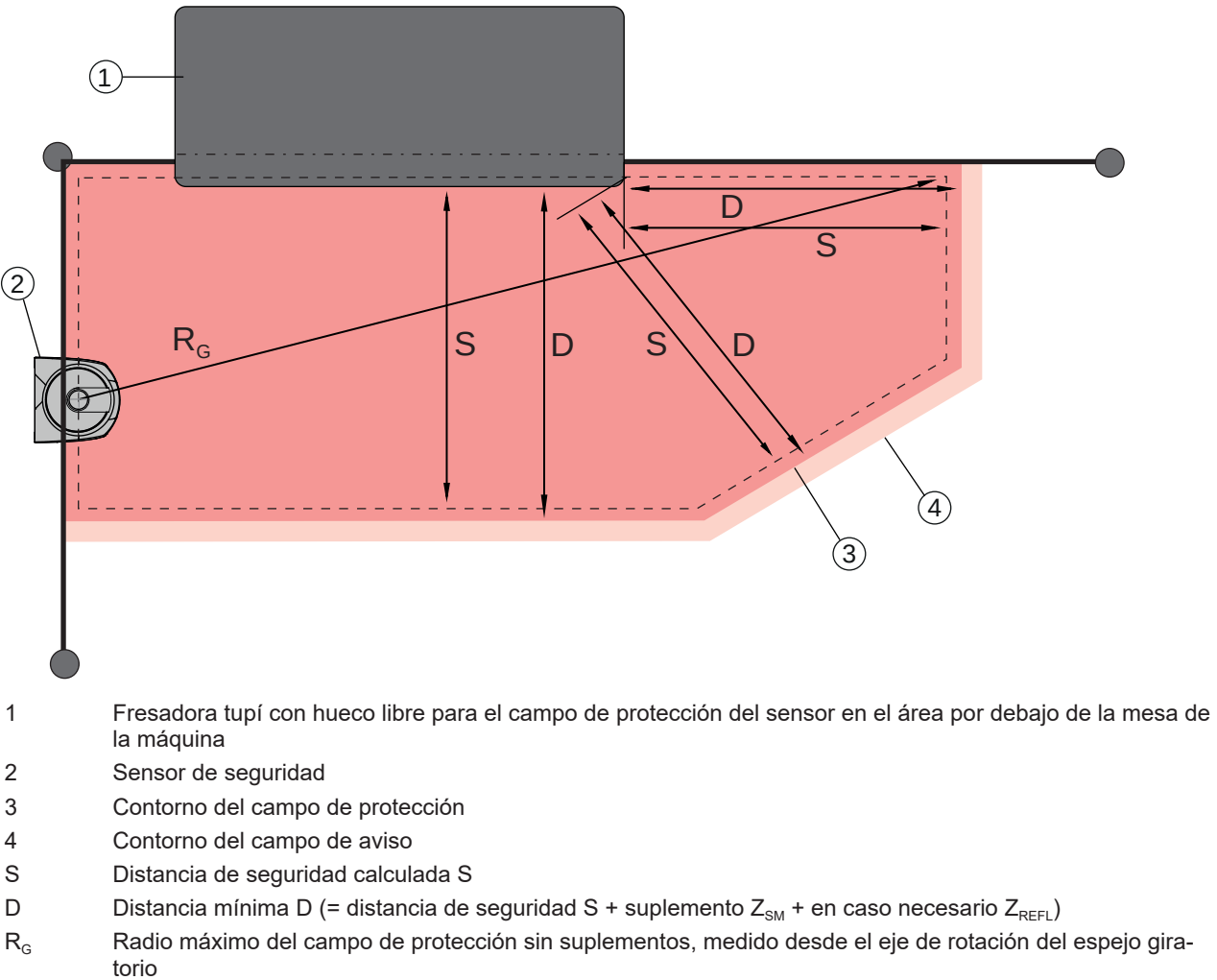
Figura 7.12: Determinación del contorno de un campo de protección horizontal fijo
