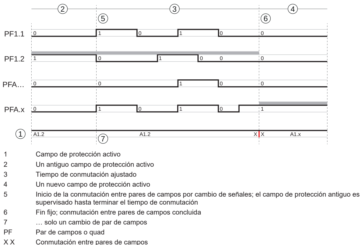
Figura 5.3: Diagrama de tiempos y señales: supervisión solapada
