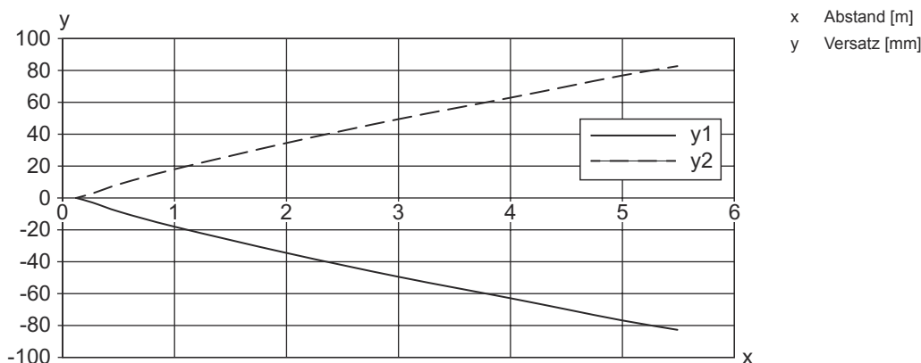
Typ. Funktionsreserve
