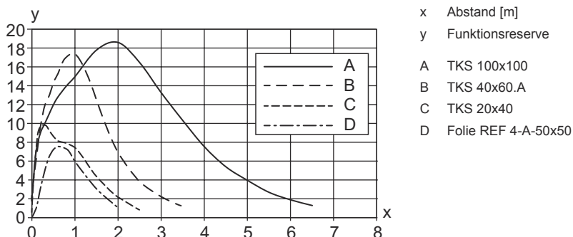
Typ. Funktionsreserve
