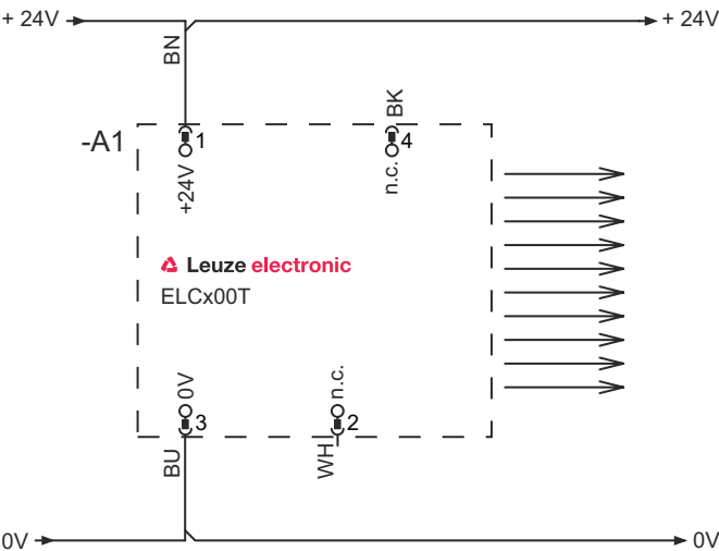
Schéma de raccordement de l'émetteur
