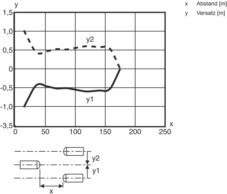
Typ. Ansprechverhalten
