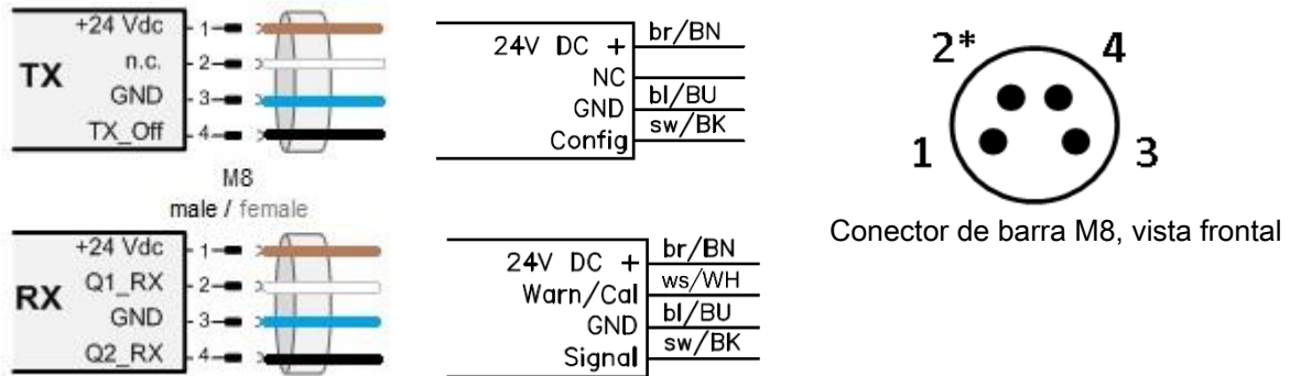
Figura 5: Modelo de conector M8, final de cable abierto
