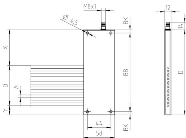
Figura 7: CSL 505 con distancia entre haces de 5 mm
