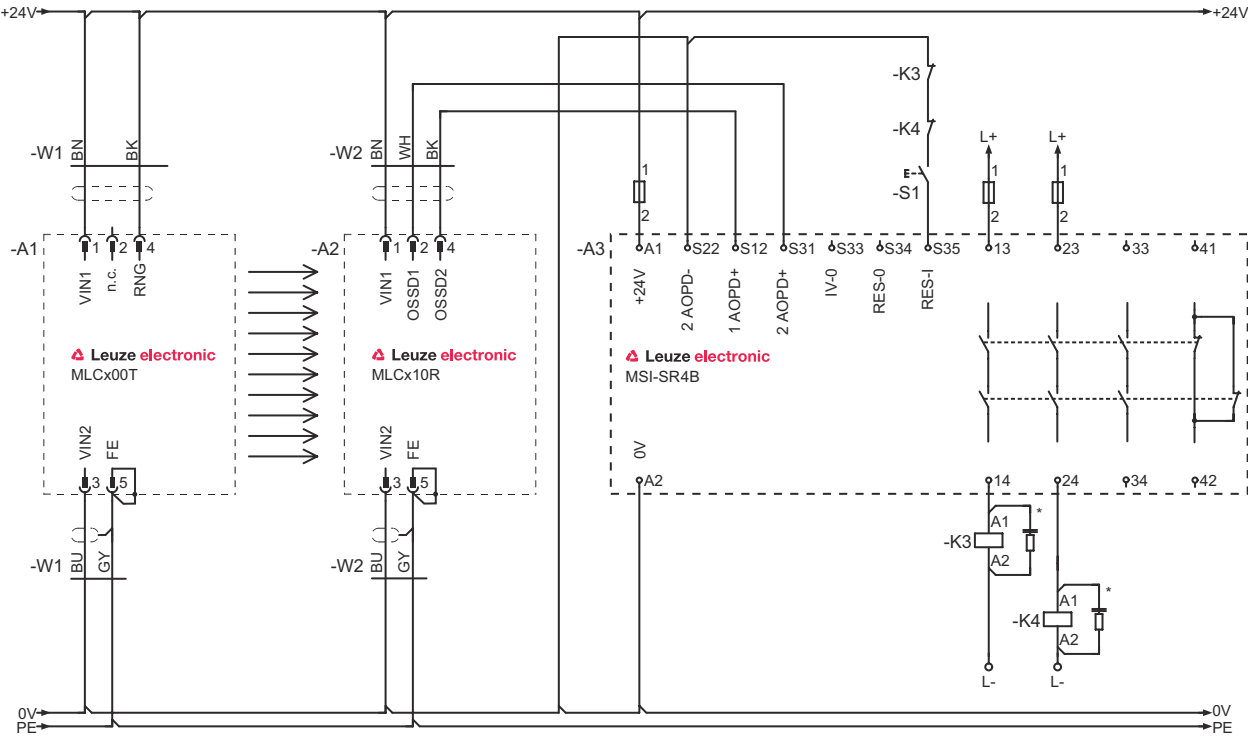
後から切り替えられる安全スイッチングデバイスMSI-SR4Bの切り替え例
