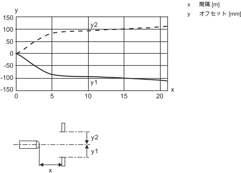
典型的な応答動作 ( TKS100x100 )
