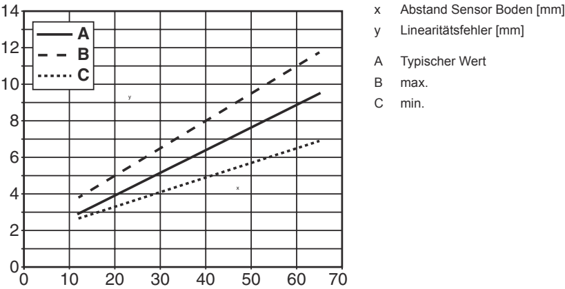
Kennlinie typischer Wert: Linearitätsfehler
