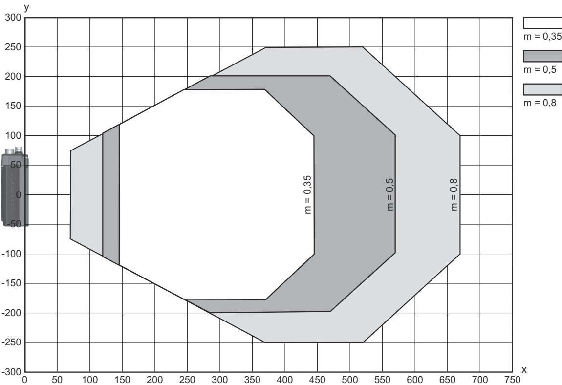
Leesveldcurve
