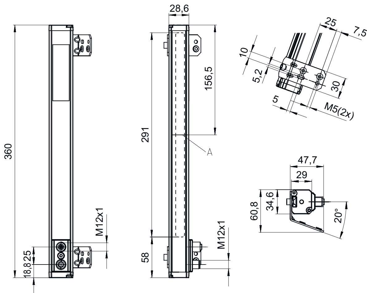
A 一体型光源
