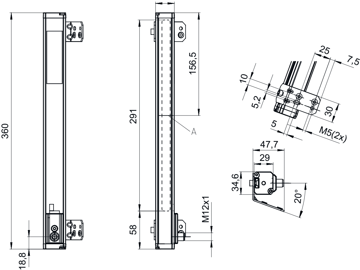
A 一体型光源
