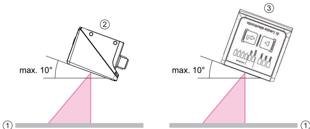
Figura 6.1: Montaggio con angolo di inclinazione frontale o laterale
