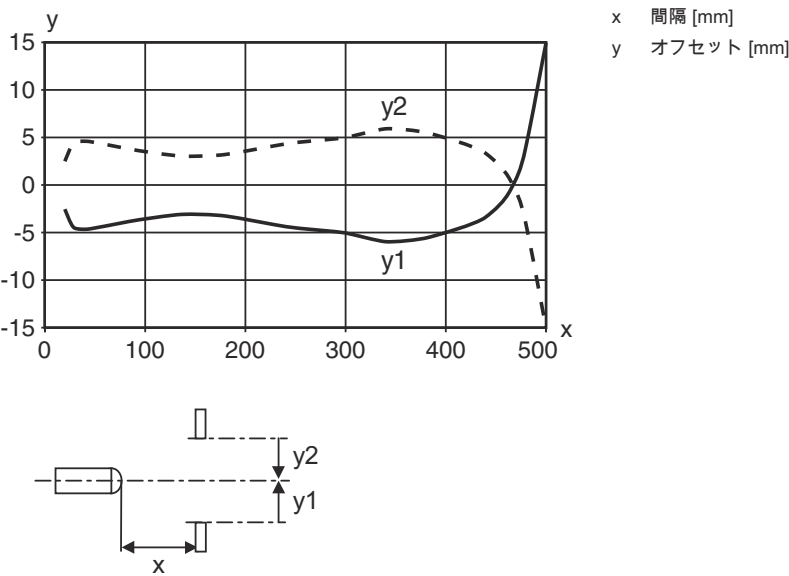
典型的応答挙動 ( 調整距離 500mm )
