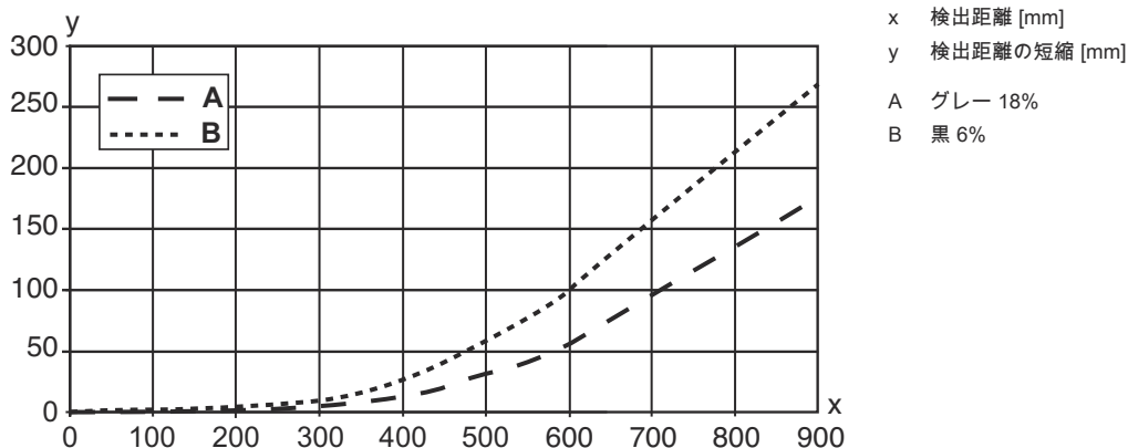
典型的な黒白動作
