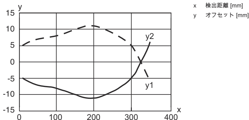
典型的応答挙動 (調整距離 350mm)
