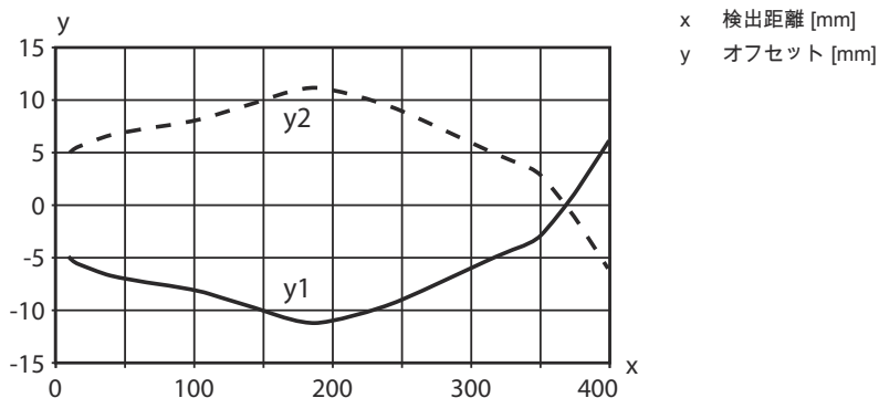
典型的応答挙動 (調整距離 400mm)
