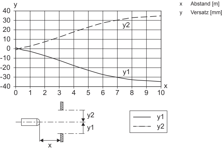
Typ. Ansprechverhalten (TKS100x100)
