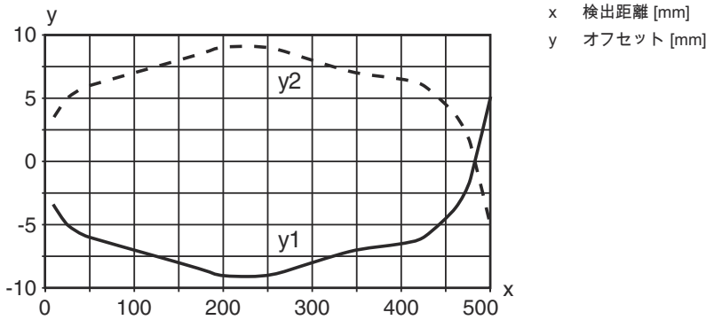
典型的応答挙動 (調整距離 500mm)
