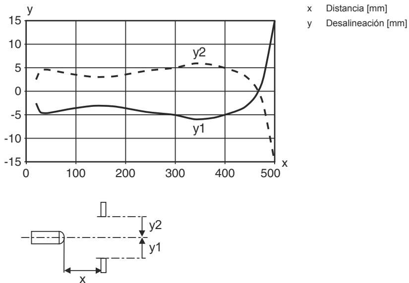
Comportamiento de respuesta típ. (distancia de ajuste 500 mm)
