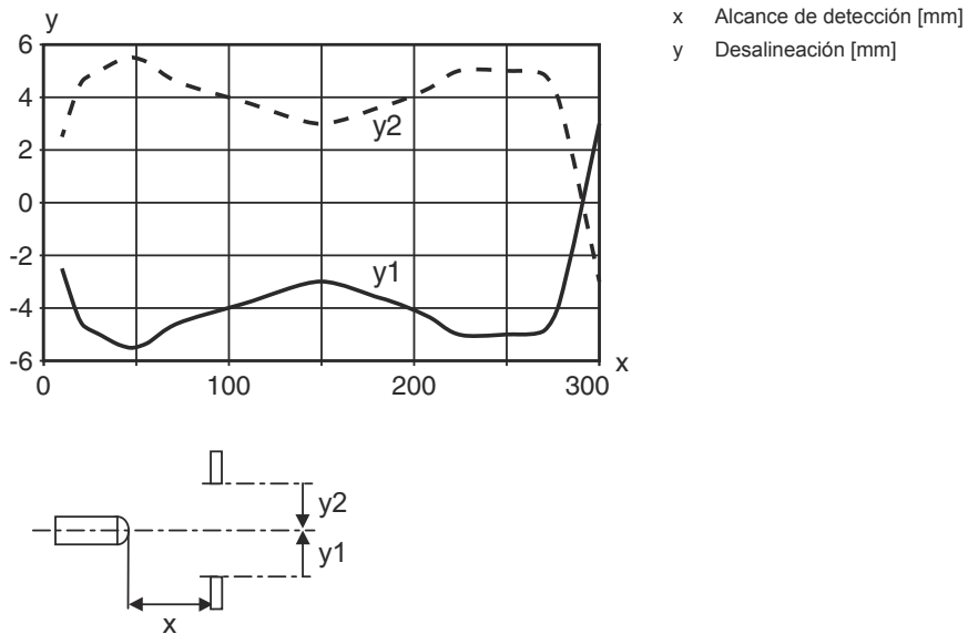
Comportamiento de respuesta típ. (distancia de ajuste 500 mm)
