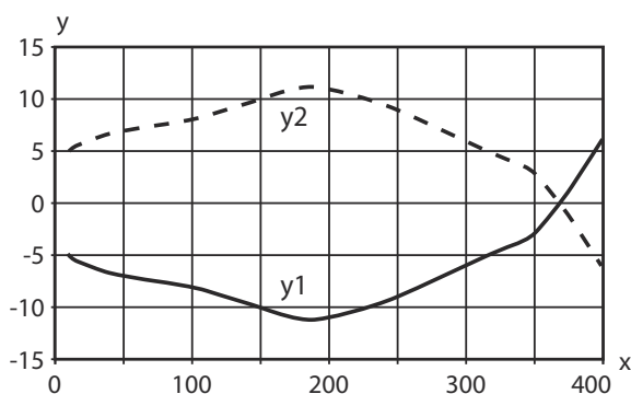
典型的応答挙動 (調整距離 400mm)
