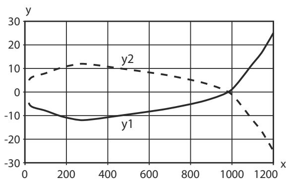
典型的応答挙動 (調整距離 1200mm)
