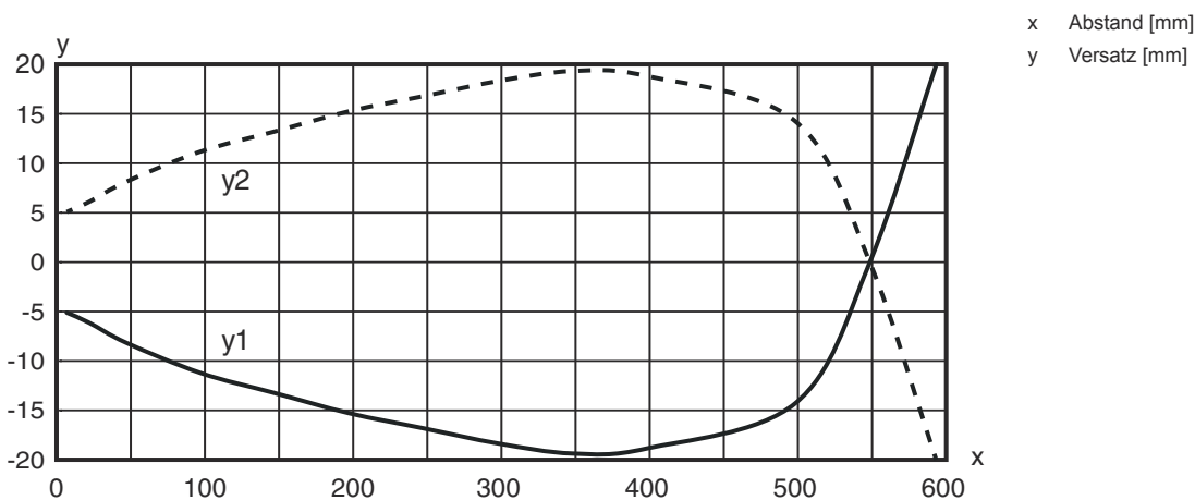
Typ. Ansprechverhalten (Einstellentfernung 600 mm)
