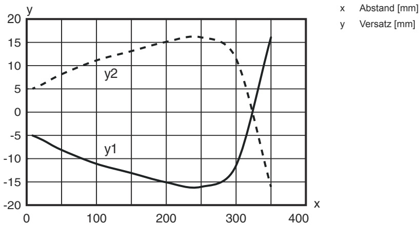
Typ. Ansprechverhalten (Einstellentfernung 350 mm)
