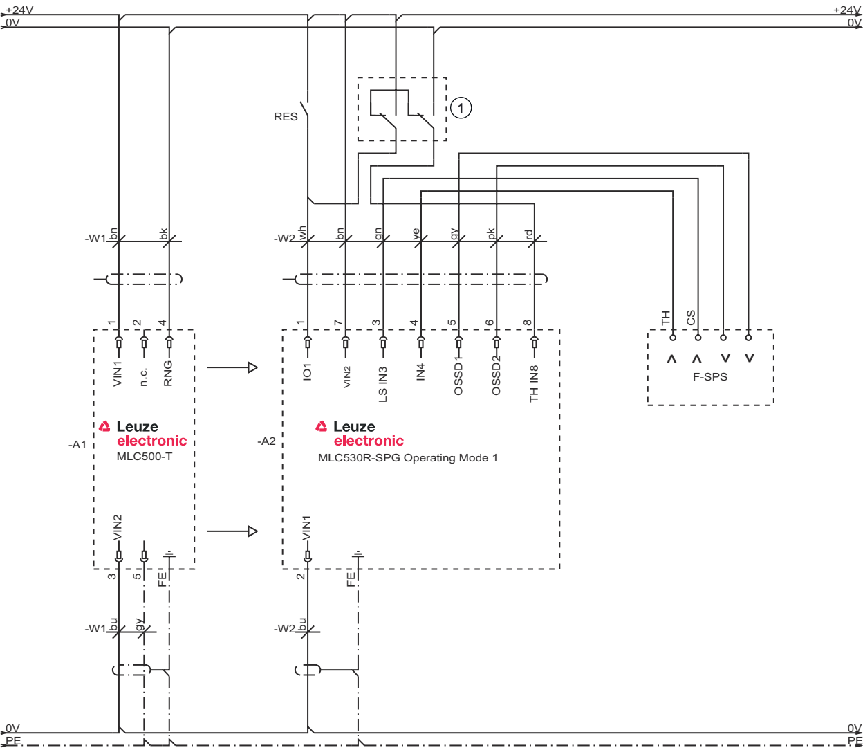
运行模式 1：含智能过程门控 (SPG) 的连接示范
