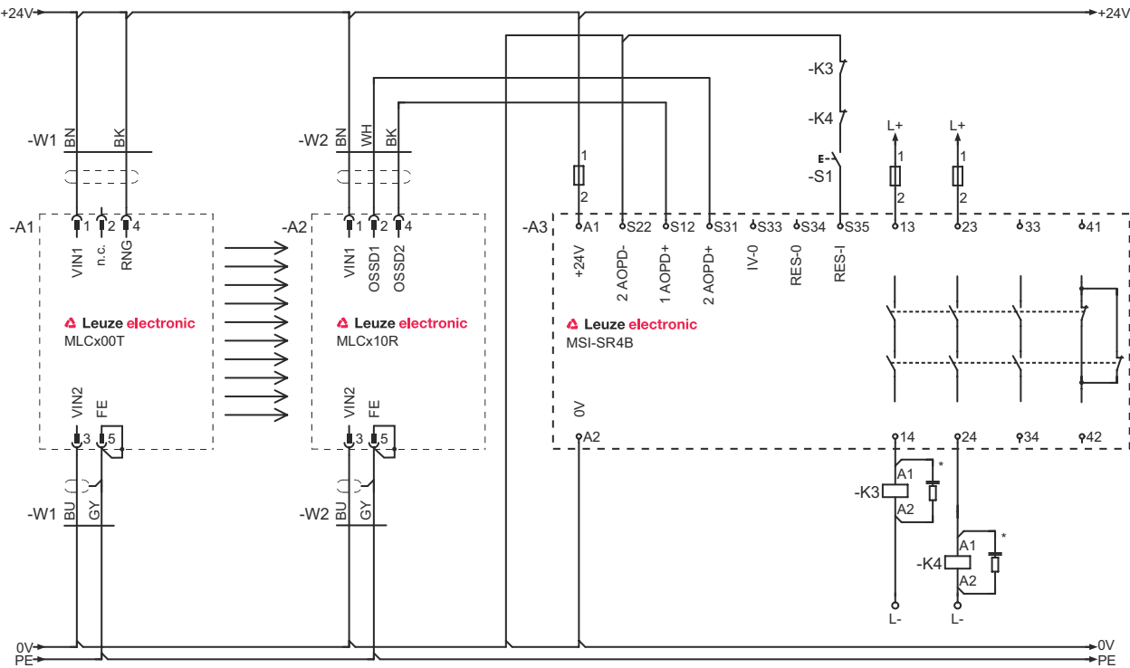
带后置安全控制器MSI-SR4B的接线示例
