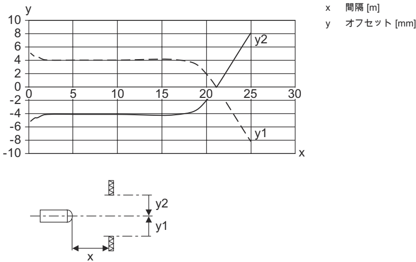
典型的な応答動作 ( TKS100x100 )
