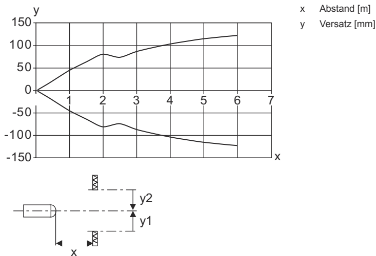
Typ. Funktionsreserve
