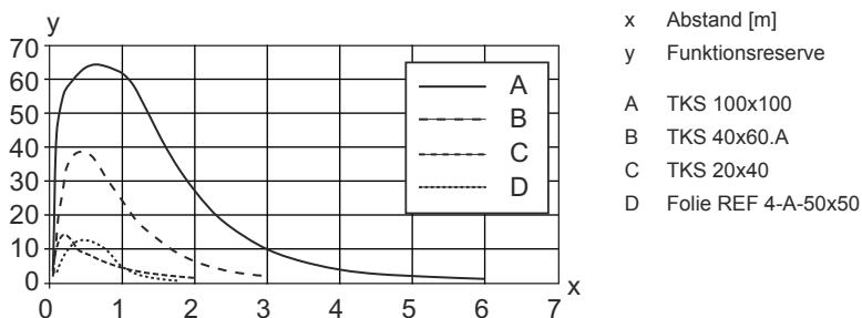
Typ. Funktionsreserve
