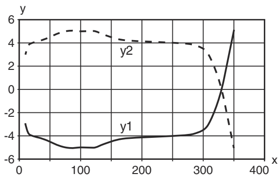
Réaction typ. (distance de réglage 350 mm)
