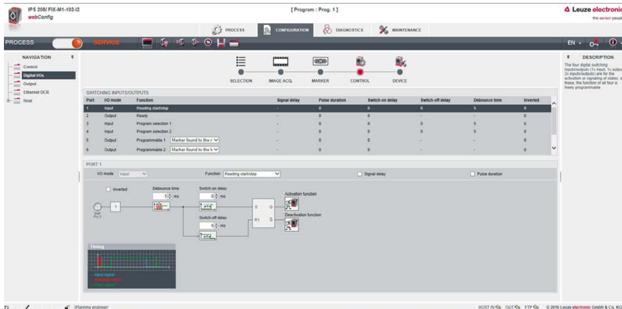
图 9.8: 数字 IO
