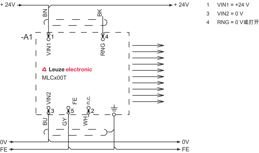
传输通道C1，标准有效范围
