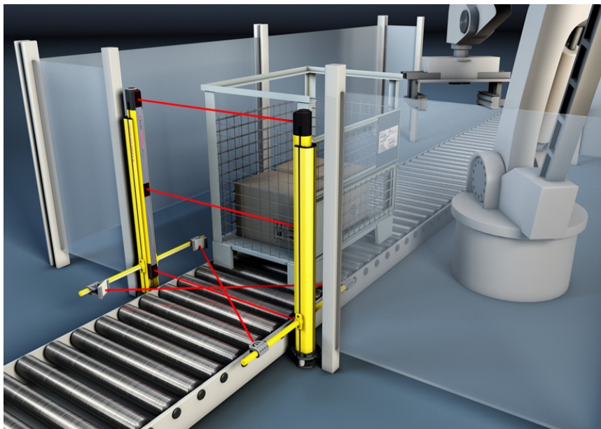
图 5.2: 在码堆机器人应用中使用收发器系统进行 3 光束防护
