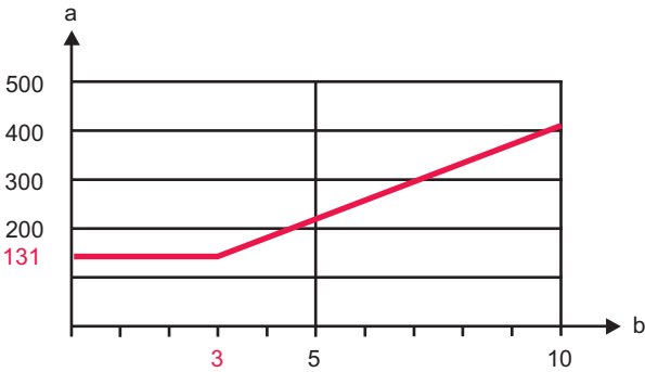
图 6.3: 根据保护区域的宽度决定的与反射平面的最小距离
