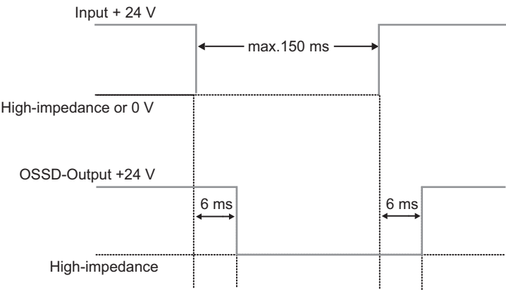
图 4.1: MLD 312 OSSD 开关量输出对于一个外部测试要求的反应
