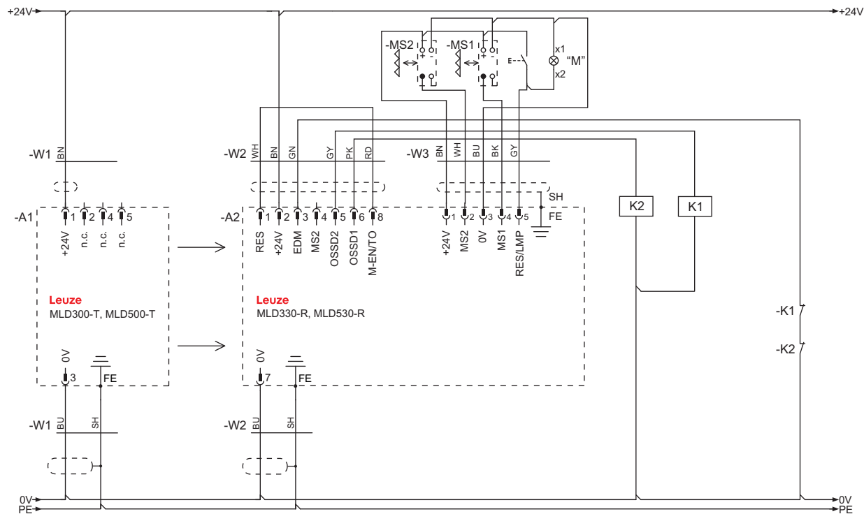
图 7.13: 连接示例 MLD 330, MLD 530 ( 发射器 - 接收器系统 ) : 定时控制的 2 个传感器屏蔽 , 100 小时屏蔽超时 ( 收发器连接与此类同 )
