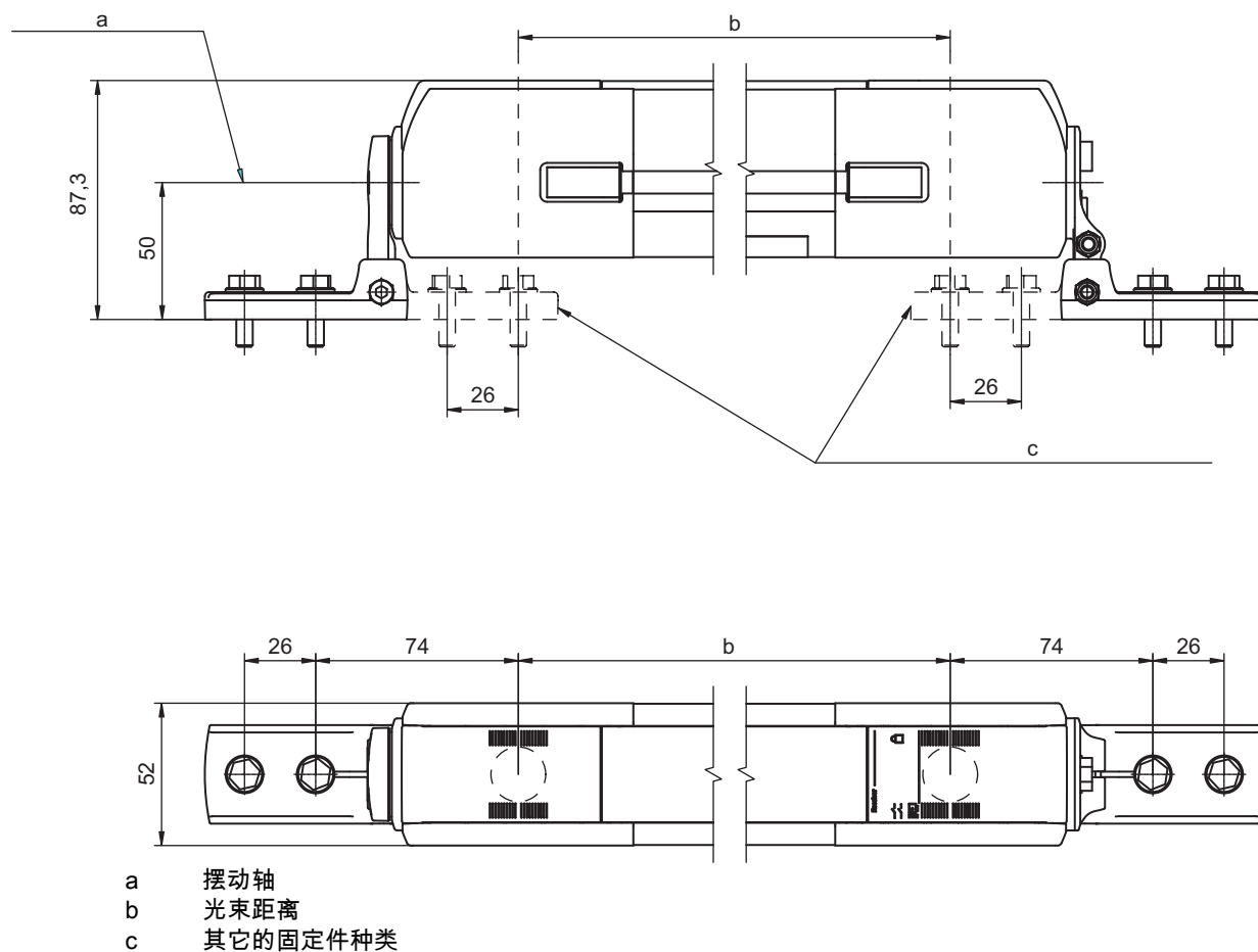
图 14.11: BT-240B, BT-240C 的安装尺寸
