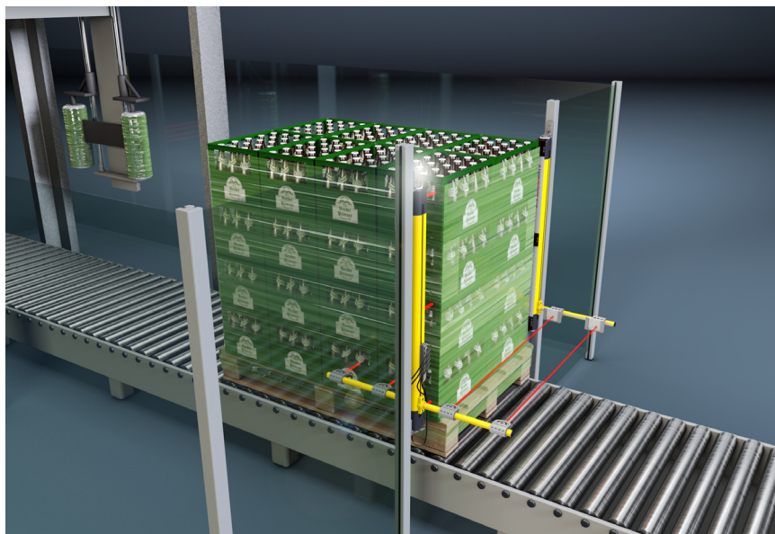
图 5.4: 用于输送辊道的带定时控制 4 个传感器屏蔽的出入口保护装置 (MLD 535, 预装屏蔽传感器套件)
