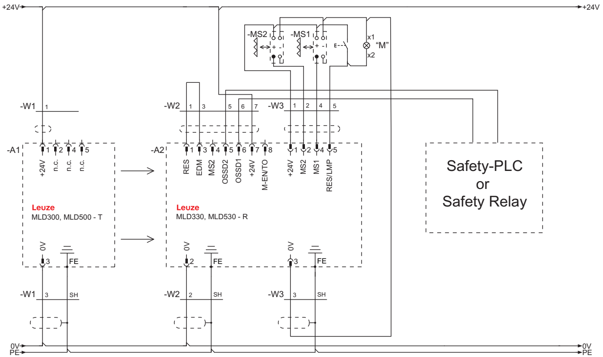
图 7.18: 连接示例 MLD 330, MLD 530 ( 发射器 - 接收器系统 ) : 局部屏蔽 ( 收发器连接与此类同 )
