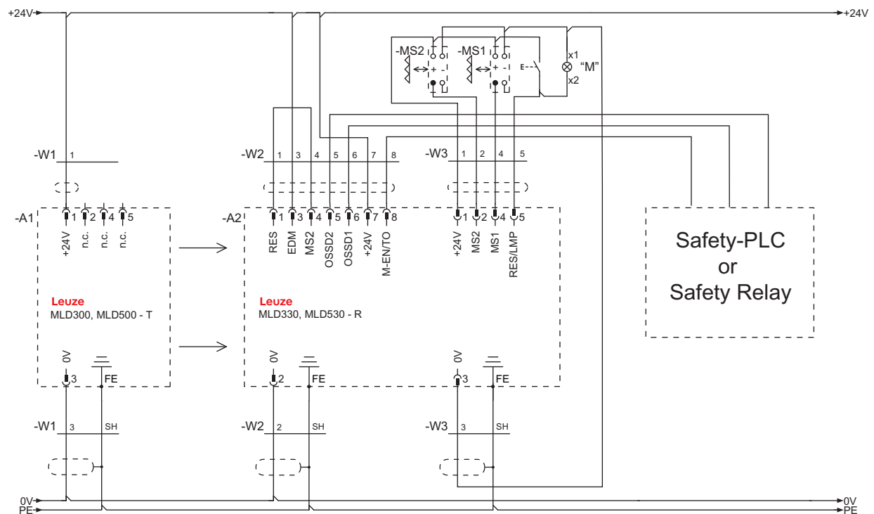
图 7.17: 连接示例 MLD 330, MLD 530 (发射器 - 接收器系统): 屏蔽使能 (收发器连接与此类同)
