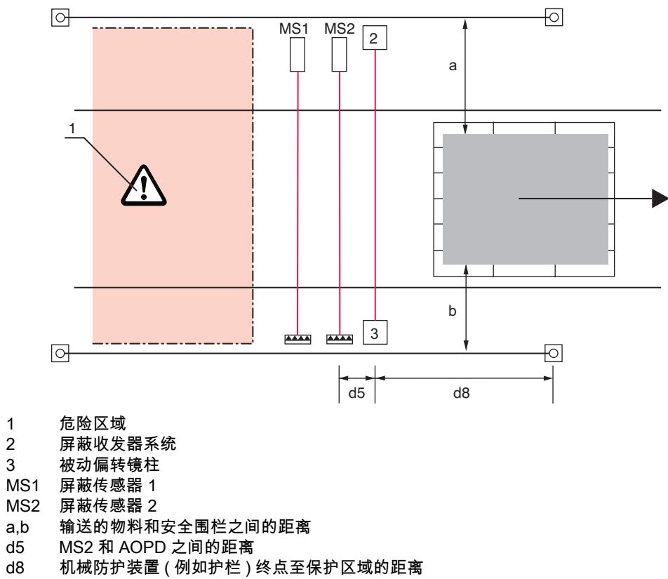
图 6.10: 顺序控制 2 个传感器屏蔽情况下屏蔽传感器的典型安装位置 ( 示例参照 IEC 62046 )
