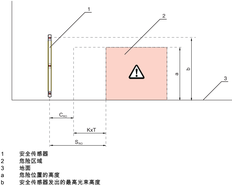
图 6.2: 有爬行或跨越进入可能性时的安全距离的附加值
