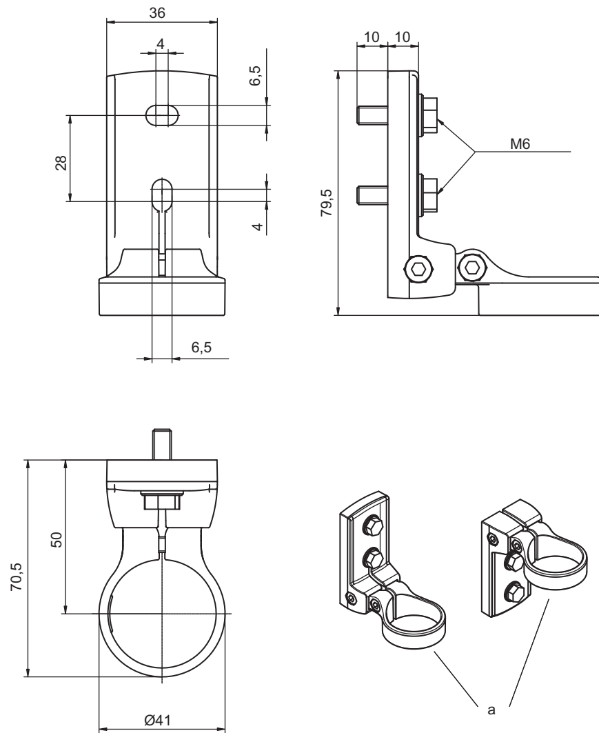
图 14.10: 转动支架 BT-240C
