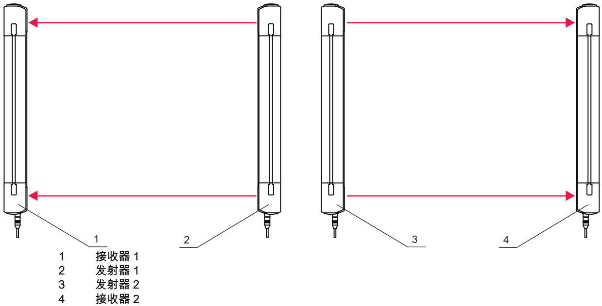
图 6.7: 对立位置的安装
