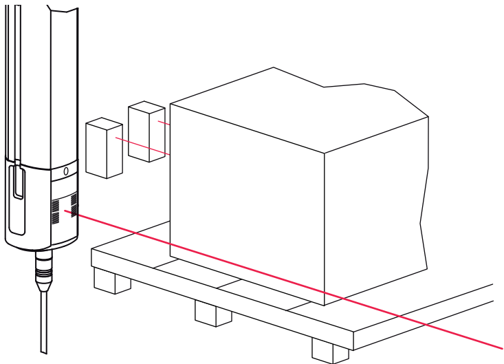
图 6.11: 屏蔽传感器高度的定位
