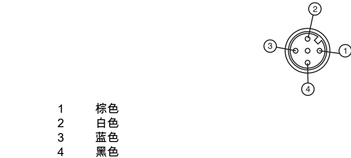
图 7.1: MLD 300、MLD 500 发射器插头引脚配置
