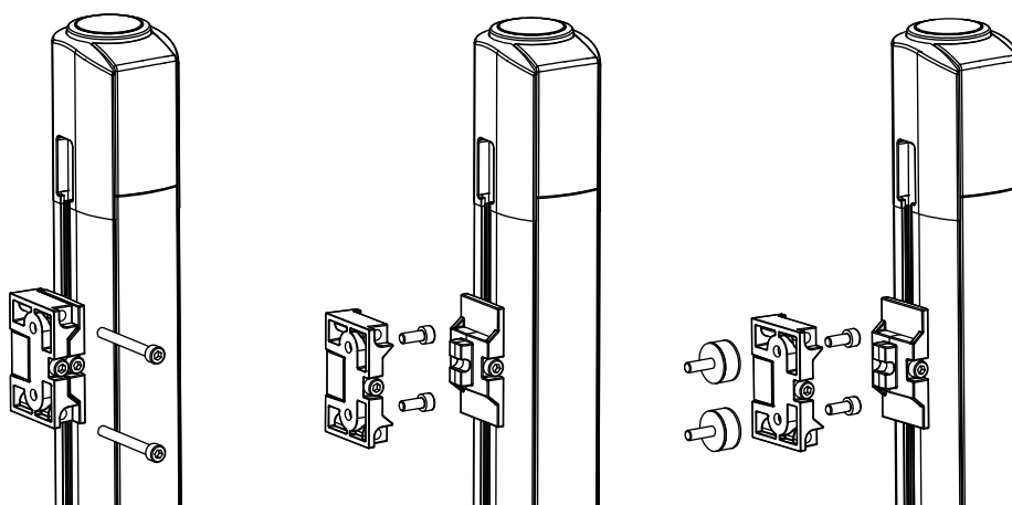
图 6.16: 夹紧旋转固定器 BT-2SB10
