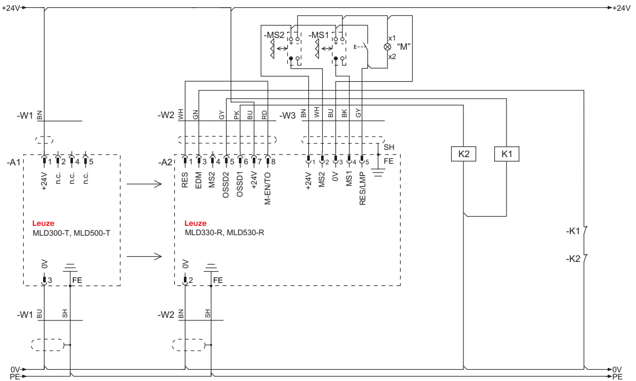
图 7.15: 连接示例 MLD 330, MLD 530 ( 发射器 - 接收器系统 ) : 顺序控制的 2 个传感器屏蔽 ( 收发器连接与此类同 )
