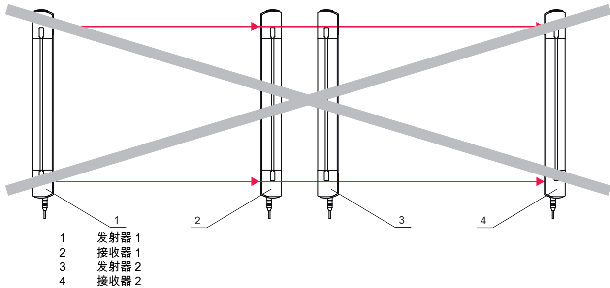
图 6.6: 由于错误的安装导致相邻安全传感器的光学串扰
