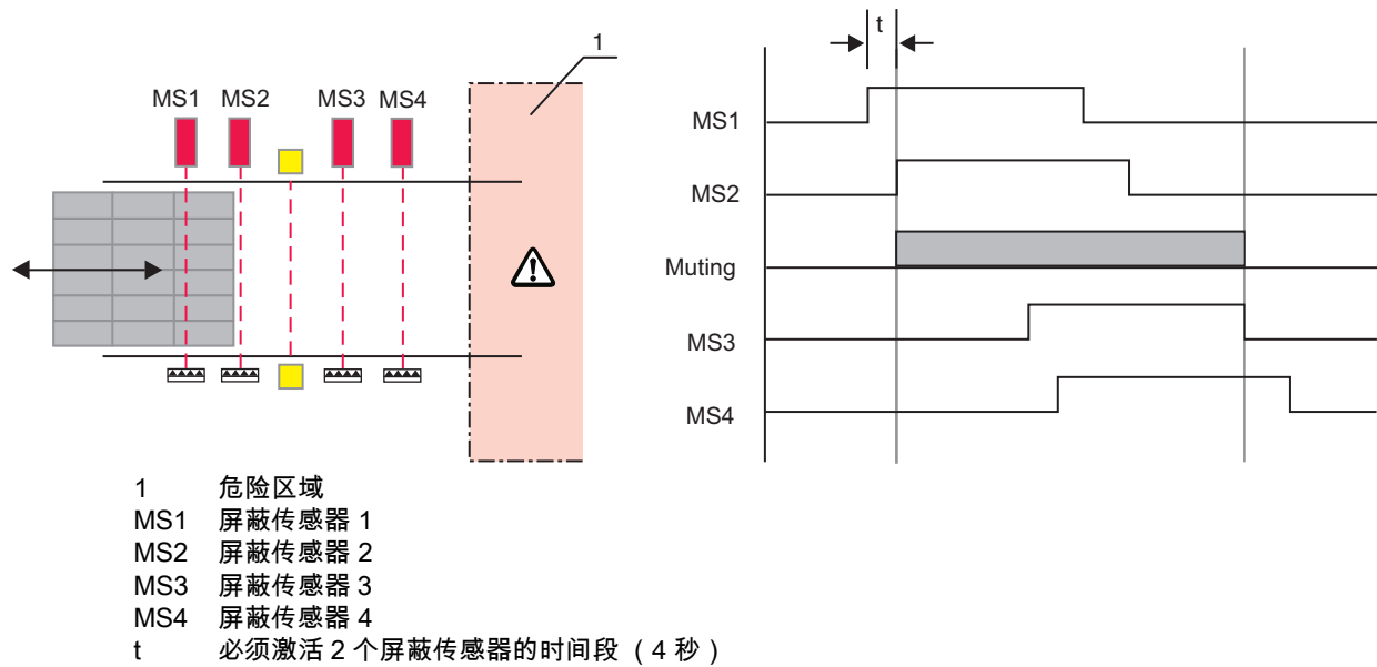
图 4.5: 定时控制的 4 个传感器屏蔽 – 屏蔽传感器的安装位置和时间过程
