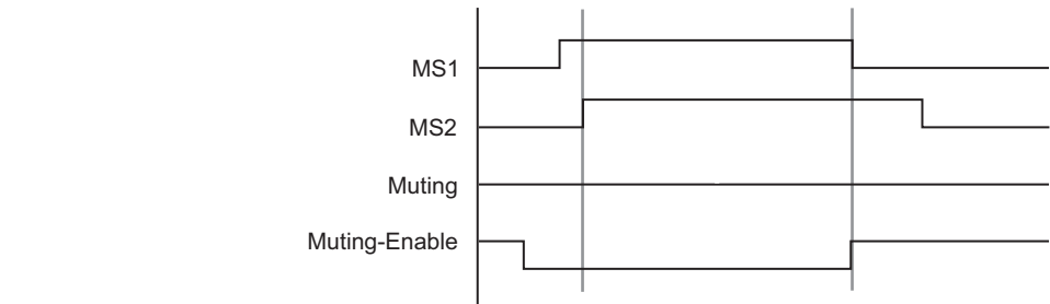
图 4.10: 没有有效的屏蔽启用信号
