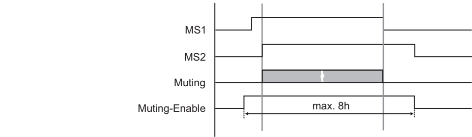
图 4.9: 屏蔽使能
