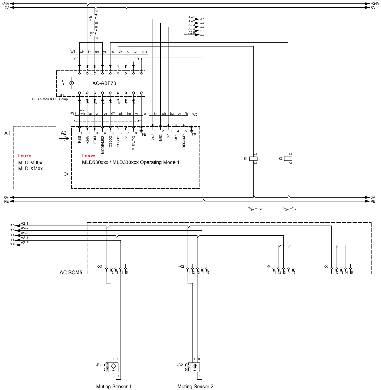
图 7.11: MLD 330, MLD 530 收发器系统的连接示例：定时控制的 2 个传感器屏蔽，屏蔽超时 10 min
