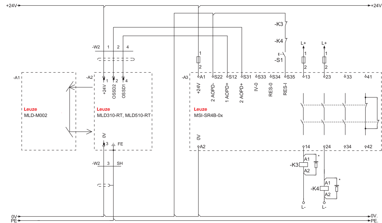
图 7.8: 连接示例 MLD 510 ( 收发器系统 ) , 带 EDM , RES 在安全继电器 MSI-SR4B-0x 内
