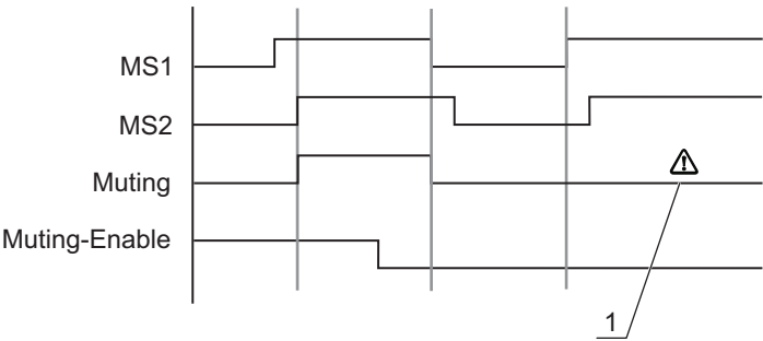
1 在此无屏蔽可能！ 图 4.11: 举例：屏蔽启用电缆上的错误
