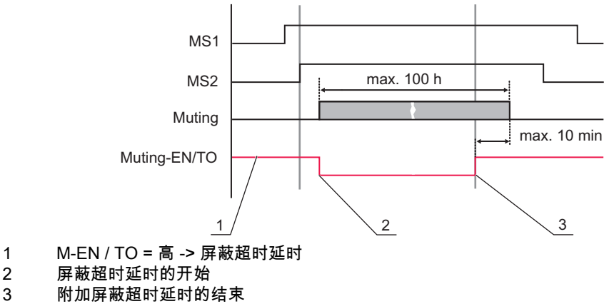
图 4.6: 屏蔽超时延时
