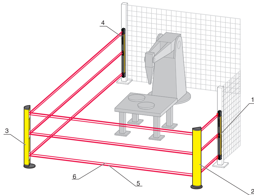
图 8.1: 借助于内置激光校准仪建立一个多向出入口保护装置。发射器最好安装在距离偏转镜柱最近的位置上。
