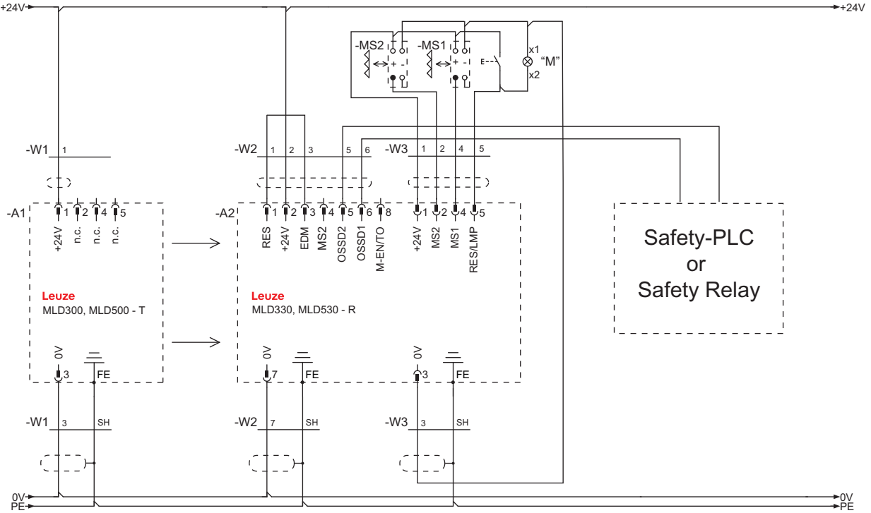
图 7.16: 连接示例 MLD 330, MLD 530 ( 发射器 - 接收器系统 ) : 顺序控制的 2 个传感器屏蔽 , 100 小时屏蔽超时 ( 收发器连接与此类同 )
