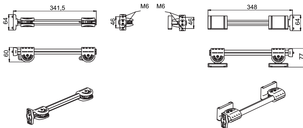
图 14.16: 屏蔽传感器套件，定时控制的 4 个传感器屏蔽
