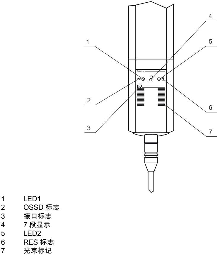
图 3.5: MLD 330, MLD 335, MLD 530, MLD 535 接收器的 7 段显示器
