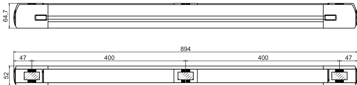
图 14.8: MLD-M 尺寸 , 3 束光偏转镜
