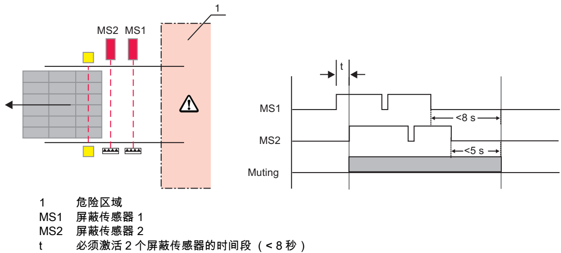
图 4.3: 顺序控制的 2 个传感器屏蔽 – 屏蔽传感器的安装位置和时间过程
