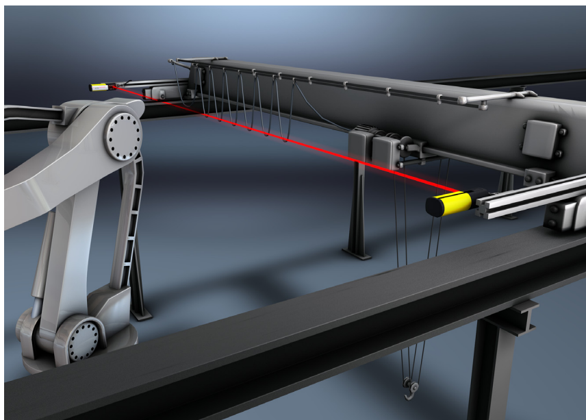
图 5.5: 单光束安全传感器通过探测机器人运动进行碰撞保护
