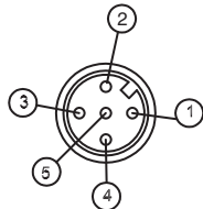
图 7.6: 插头引脚配置 MLD 500/AS-i ( 发射器，接收器 / 收发器，用于外部屏蔽指示灯的连接插口 )
