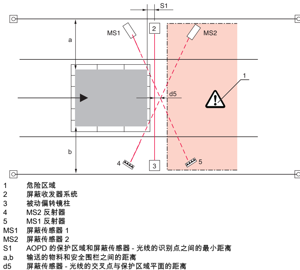
图 6.8: 使用定时控制的 2 个传感器屏蔽时，屏蔽传感器的典型安装位置（示例参照 IEC 62046）
