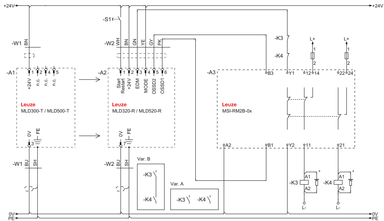
图 7.9: 连接示例 MLD 320 , MLD 520 ( 发射器 - 接收器系统 ) 和 MSI-RM2B-0x , 带 EDM 和 RES ( 收发器连接与此类同 )
