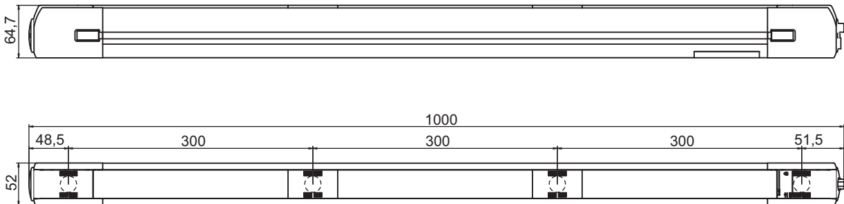
图 14.4: MLD 尺寸，4 束光束发射器，接收器
