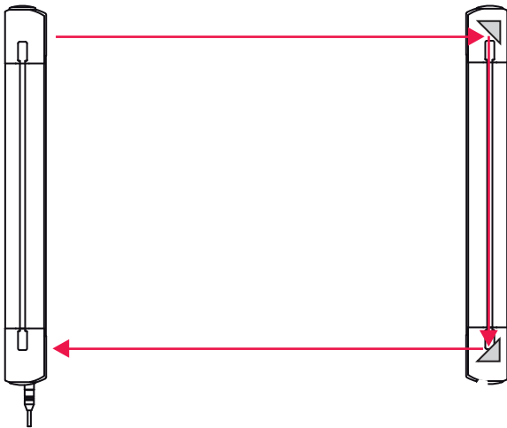
图 3.2: 收发器系统 收发器系统由一个主收发器（发射器 / 接收器）和一个被动偏转镜柱（没有电气连接，将光线偏转 2 x 90°）组成。
