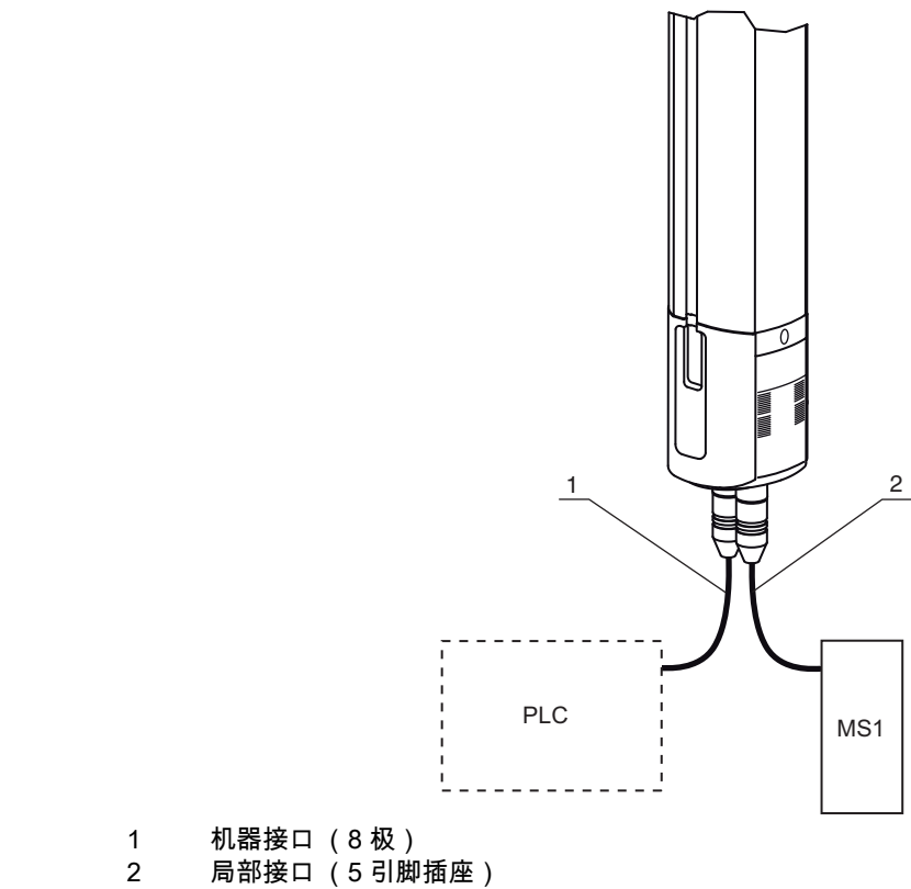
图 4.8: 2. 控制装置的屏蔽信号
