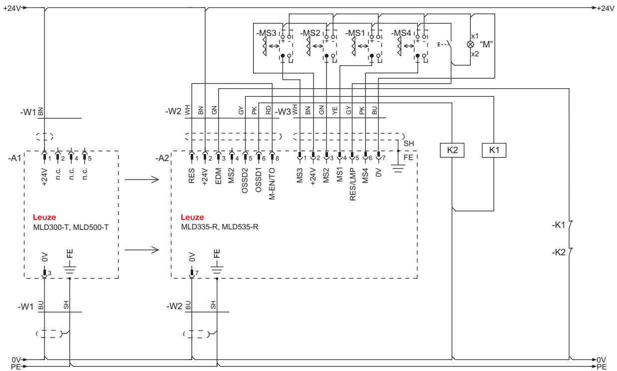
图 7.14: 连接示例 MLD 335, MLD 535 ( 发射器 - 接收器系统 ) : 定时控制的 4 个传感器屏蔽 ( 收发器连接与此类同 )
