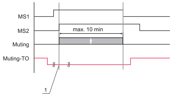
1 M-EN / TO = 低 -> 无屏蔽超时延时 图 4.7: 没有有效时间限制 - 延长的信号
