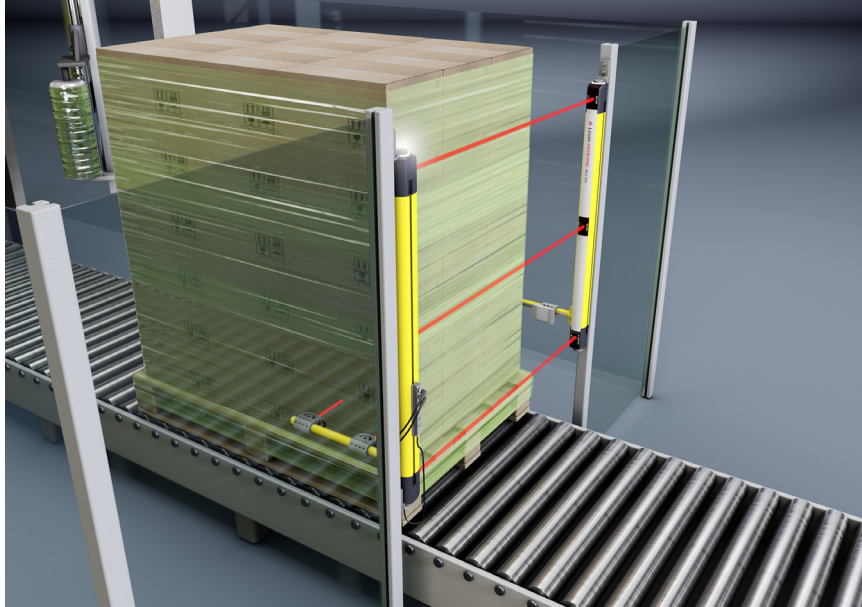
图 5.1: 从危险区域中驶出时的 3 光束防护
