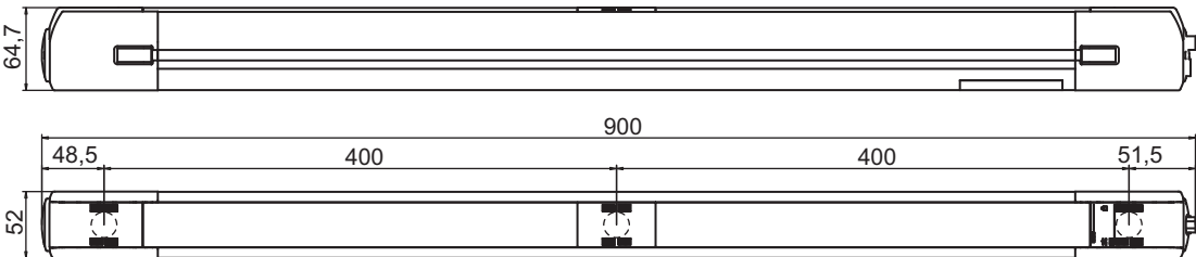
图 14.3: MLD 尺寸，3 束光束发射器，接收器
