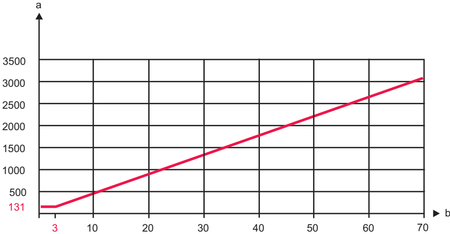
图 6.4: 根据保护区域的宽度 (最宽 10 米) 决定的与反射平面的最小距离
