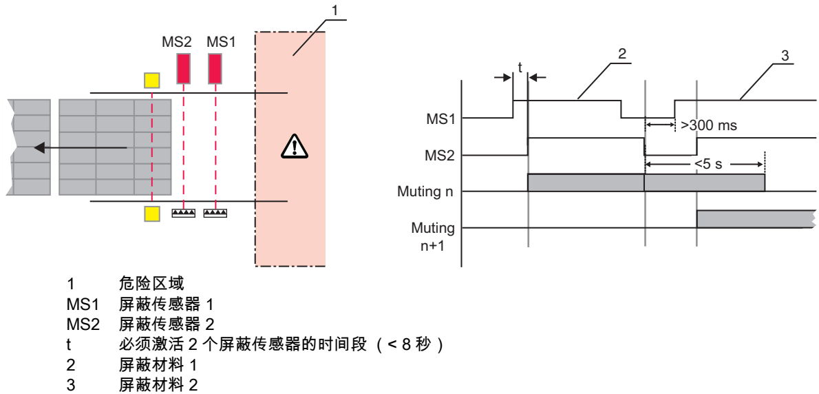
图 4.4: 密集输送序列时的屏蔽 - 屏蔽传感器的安装位置和定时
