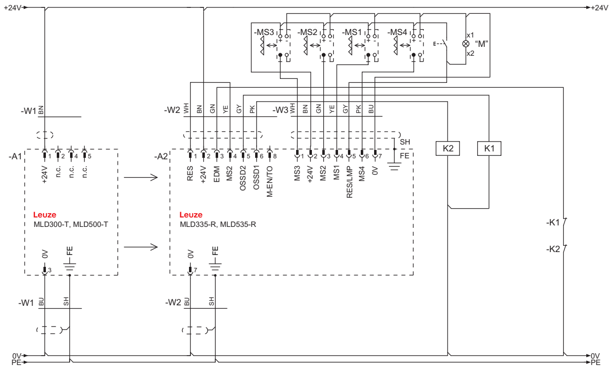
图 7.12: 连接示例 MLD 335, MLD 535 ( 发射器 - 接收器系统 ) : 定时控制的 4 个传感器屏蔽, 10 分钟屏蔽超时 ( 收发器连接与此类同 )
