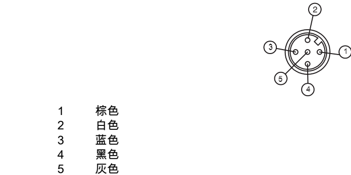
图 7.2: MLD 310、MLD 312、MLD 510 接收器插头引脚配置
