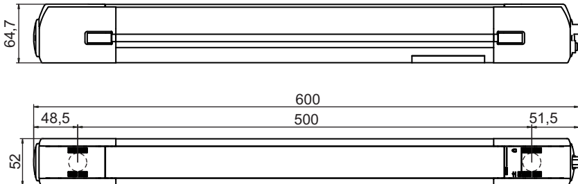
图 14.5: MLD 尺寸，2 束光束收发器
