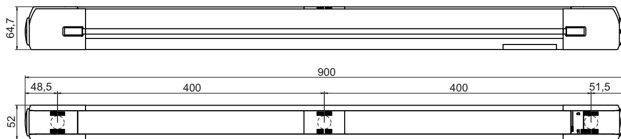
图 14.6: MLD 尺寸 , 3 束光束收发器
