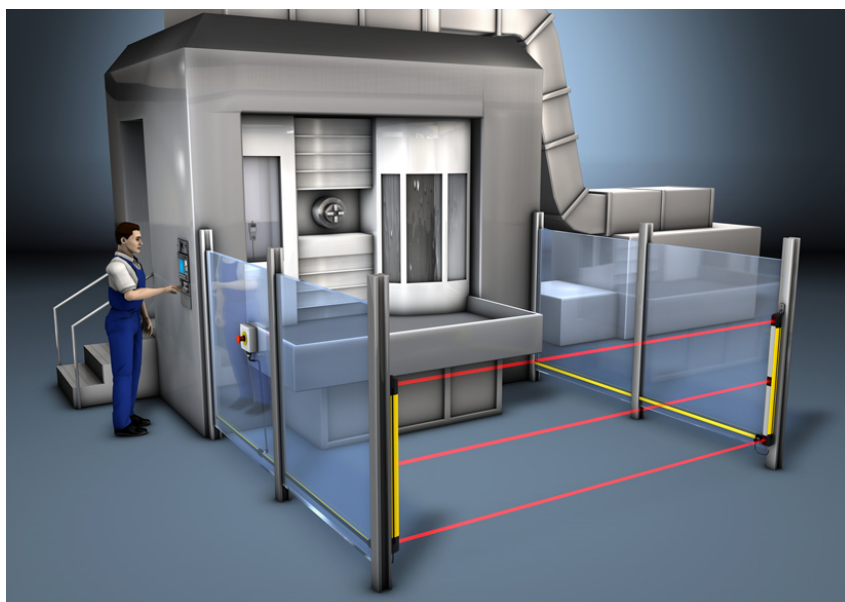
图 5.6: MLD 500/AS-i 根据 AS-i 工作安全原理的出入口保护装置，用于加工中心
