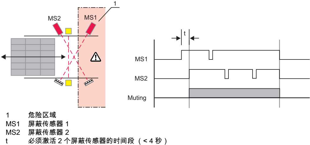
图 4.2: 定时控制的 2 个传感器屏蔽 – 屏蔽传感器的安装位置和时间过程
