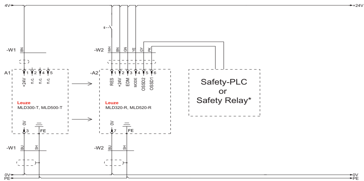
图 7.7: 连接示例 MLD 320, MLD 520 ( 发射器 - 接收器系统 ) 无 EDM , 带 RES ( 收发器连接与此类同 )
