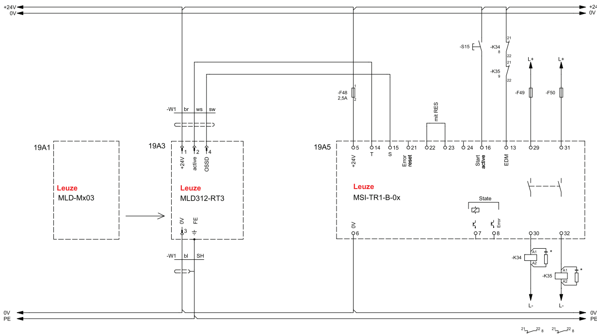
图 7.10: 连接示例 MLD 312 ( 发射器 - 接收器系统 ) 和 MSI-TR1B-0x , 带 EDM 和 RES
