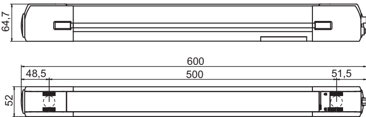
图 14.2: MLD 尺寸，2 束光束发射器，接收器
