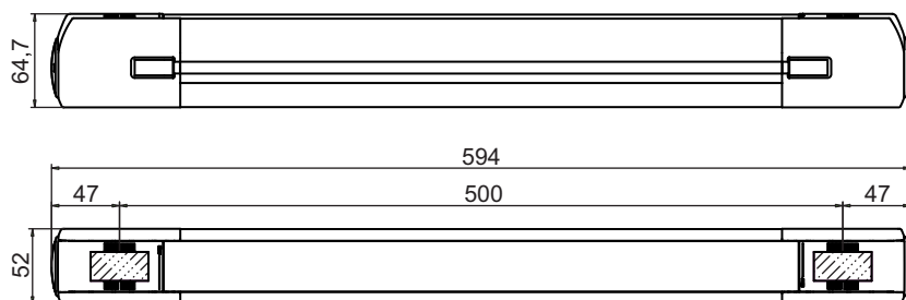
图 14.7: MLD-M 尺寸 , 2 束光束偏转镜
