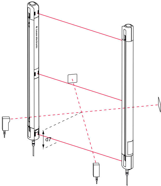
图 6.9: 屏蔽传感器在高度 d7 处的定位
