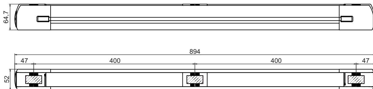
Fig. 14.8: Medidas MLD-M, espejo deflector de 3 haces
