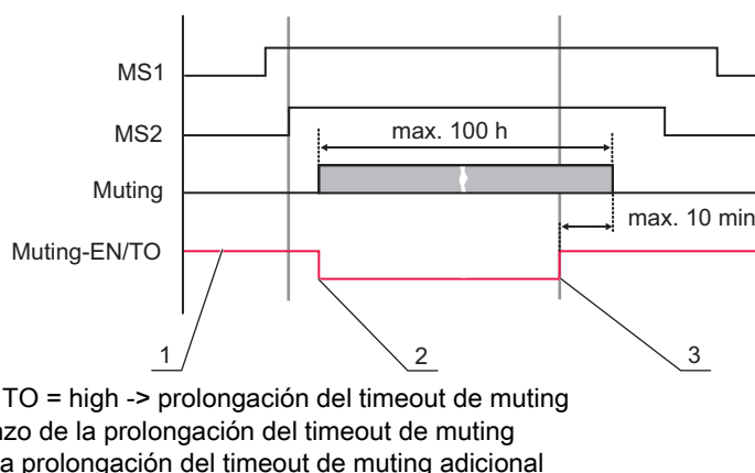
Fig. 4.6: Prolongación del timeout de muting
