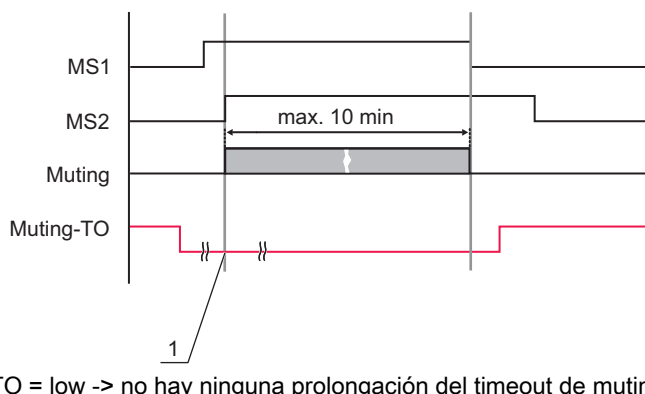
Fig. 4.7: No hay ninguna señal válida para la prolongación del timeout
