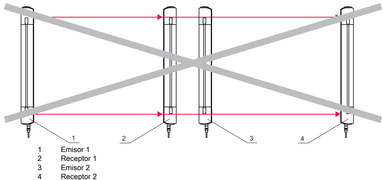
Fig. 6.6: Diafonía óptica de sensores de seguridad contiguos debido a montaje erróneo
