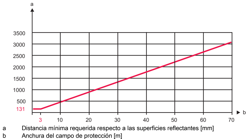
Fig. 6.5: Distancia mínima respecto a las superficies reflectantes en función de la anchura del campo de protección hasta 70 m
