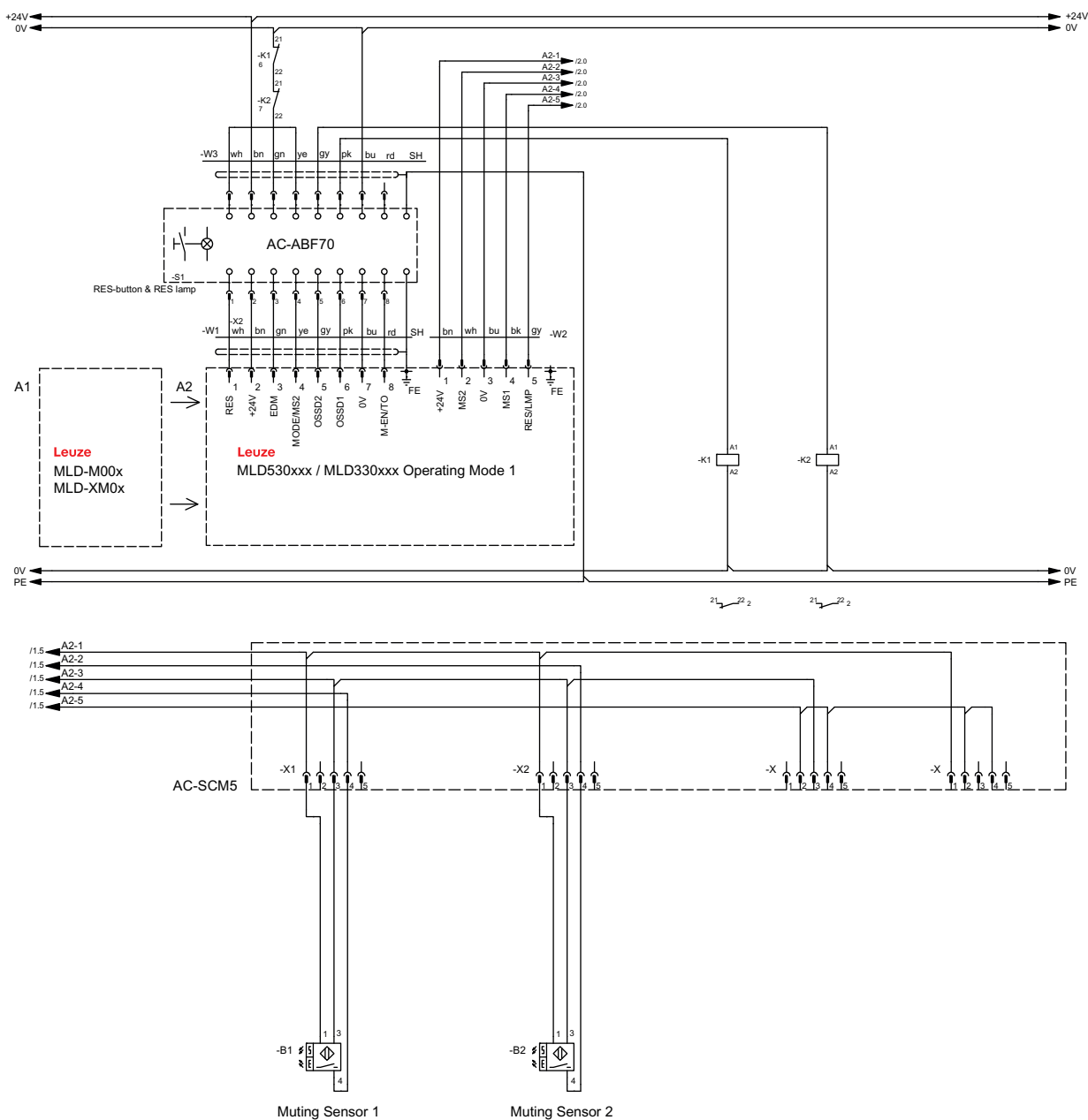
Fig. 7.11: Ejemplo de conexión del sistema transceptor MLD 330, MLD 530: muting de 2 sensores con control temporizado con timeout de muting 10 min
