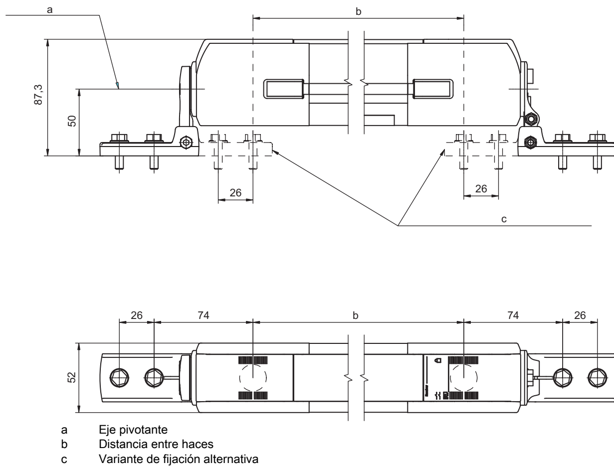
Fig. 14.11: Medidas para el montaje de BT-240B, BT-240C
