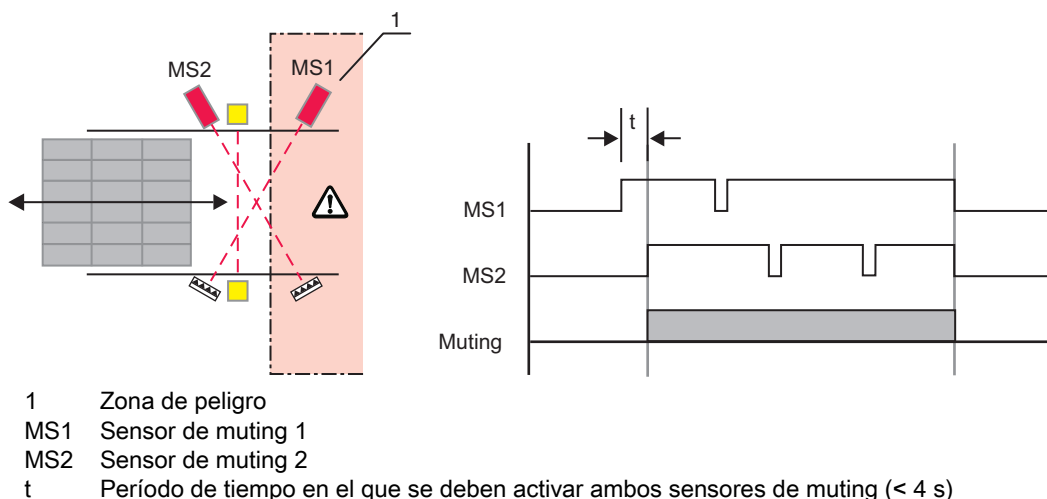
Fig. 4.2: Muting de 2 sensores con control temporizado - disposición de los sensores de muting y terminación del tiempo
