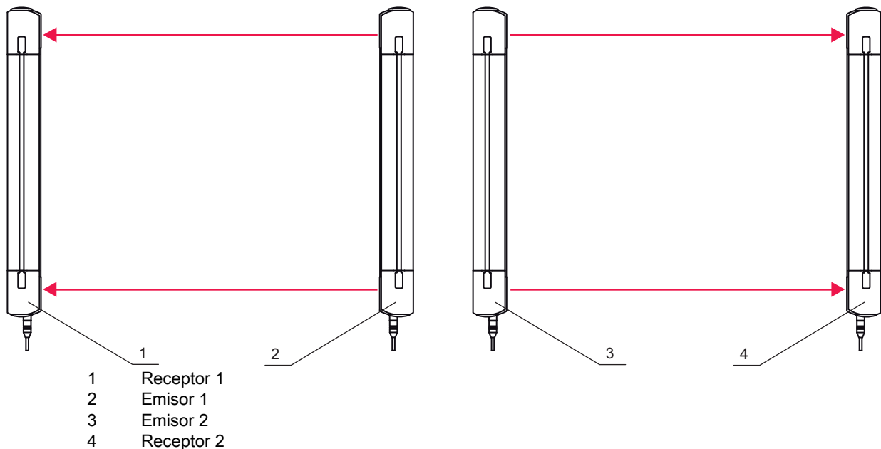
Fig. 6.7: Montaje opuesto
