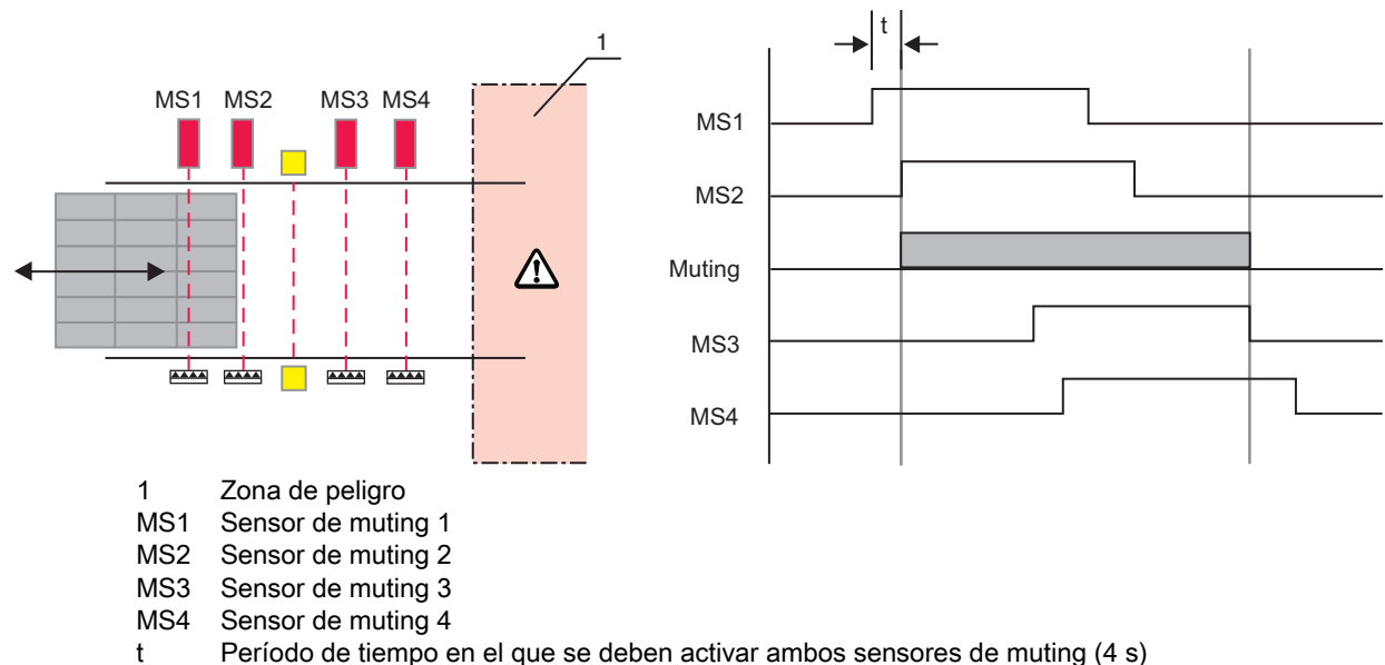
Fig. 4.5: Muting de 4 sensores con control temporizado: disposición de los sensores de muting y terminación del tiempo
