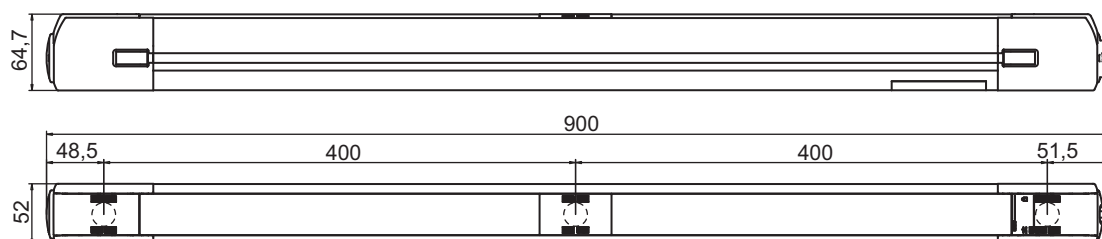
Fig. 14.3: Medidas MLD, emisor de 3 haces, receptor
