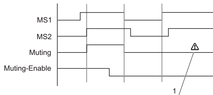
Fig. 4.11: Ejemplo: error en la línea Muting-Enable
