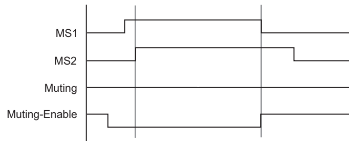
Fig. 4.10: No hay ninguna señal Muting-Enable válida
