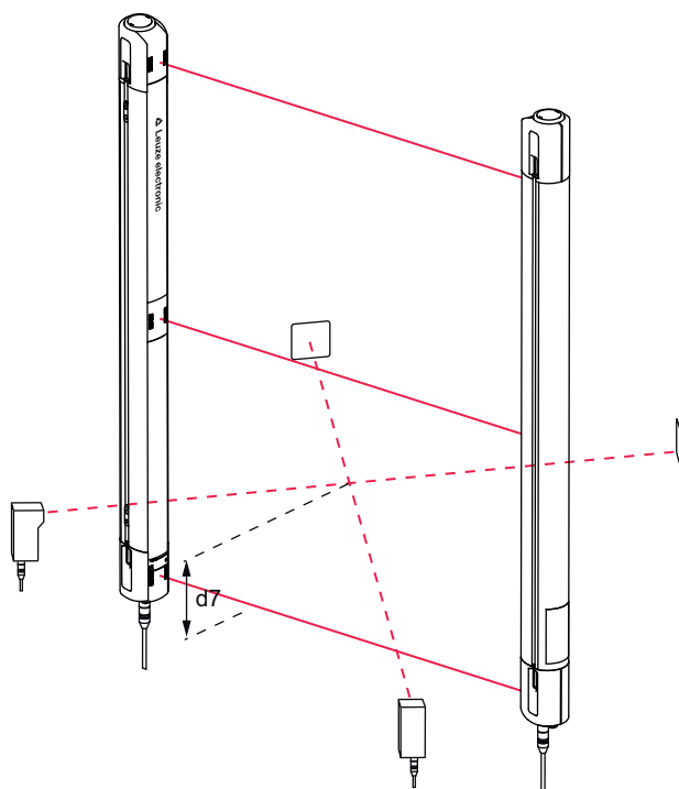
Fig. 6.9: Disposición de los sensores de muting en la altura d7
