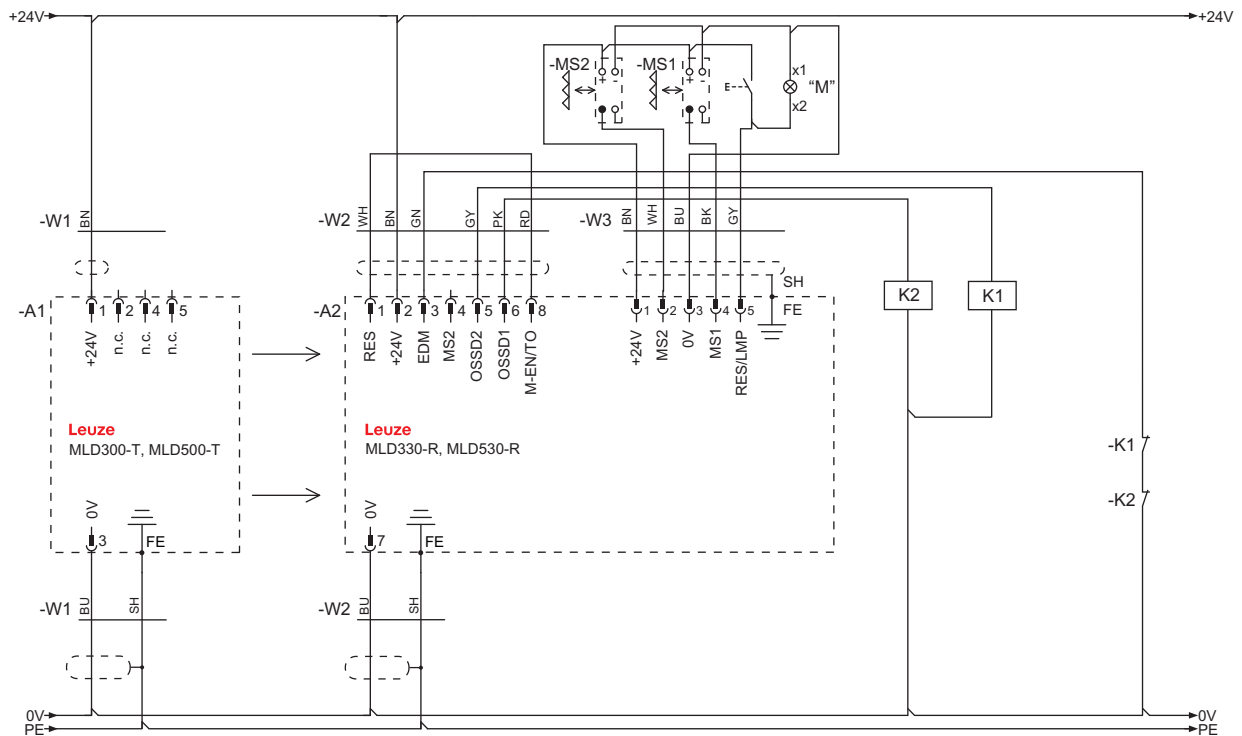
Fig. 7.13: Ejemplo de conexión MLD 330, MLD 530 (sistema emisor-receptor): muting de 2 sensores con control temporizado con timeout de muting 100 h (conexión transceptor analógico al respecto)
