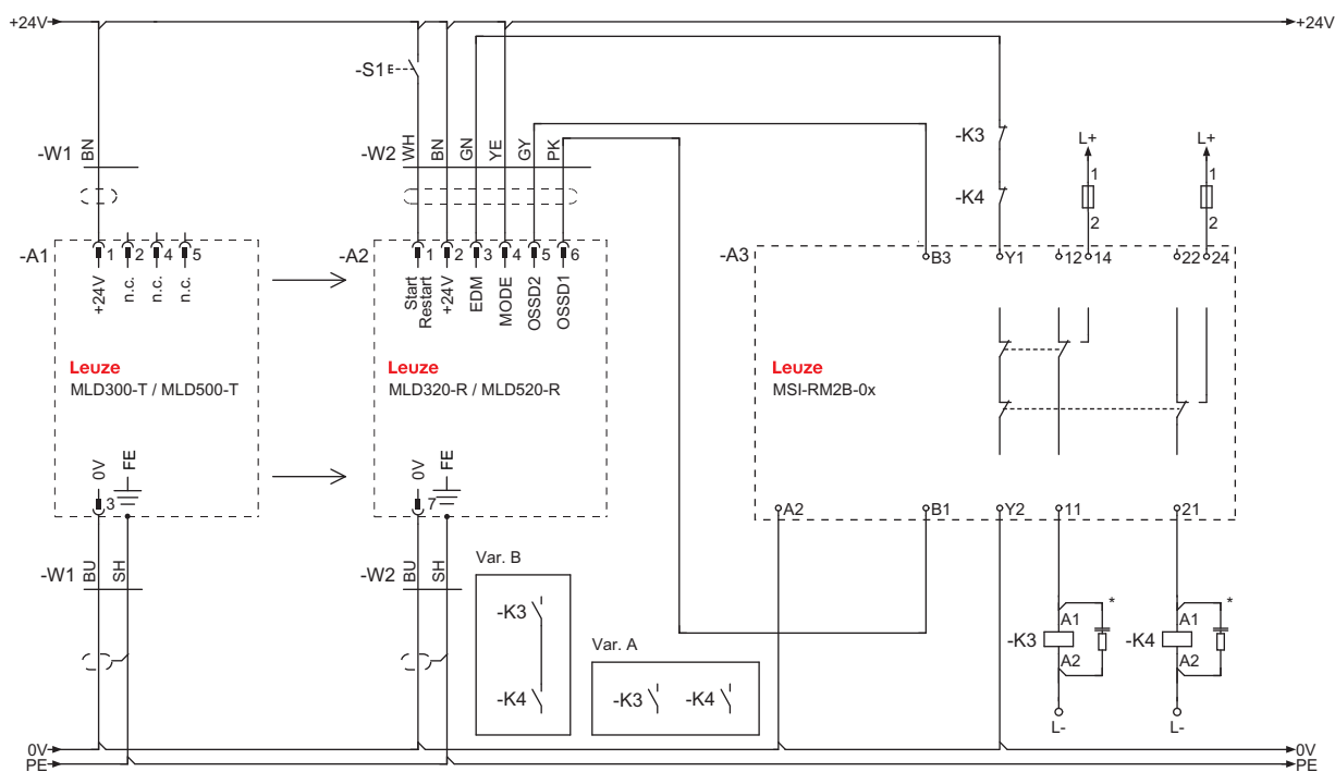
Fig. 7.9: Ejemplo de conexión MLD 320, MLD 520 (sistema emisor-receptor) y MSI-RM2B-0x, con EDM y RES (conexión transceptor analógico al respecto)
