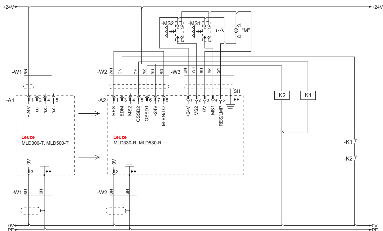
Fig. 7.15: Ejemplo de conexión MLD 330, MLD 530 (sistema emisor-receptor): muting de 2 sensores con control secuencial (conexión transceptor analógico al respecto)
