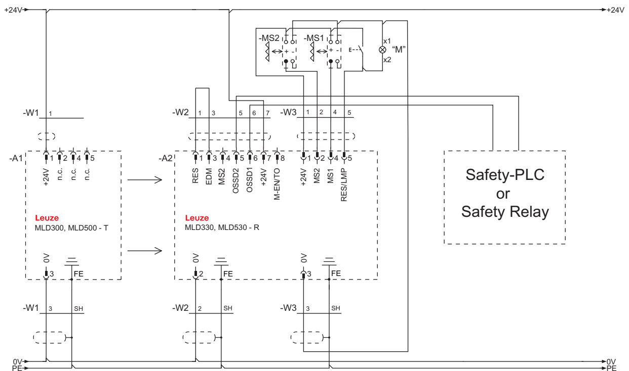
Fig. 7.18: Ejemplo de conexión MLD 330, MLD 530 (sistema emisor-receptor): muting parcial (conexión transceptor analógico al respecto)
