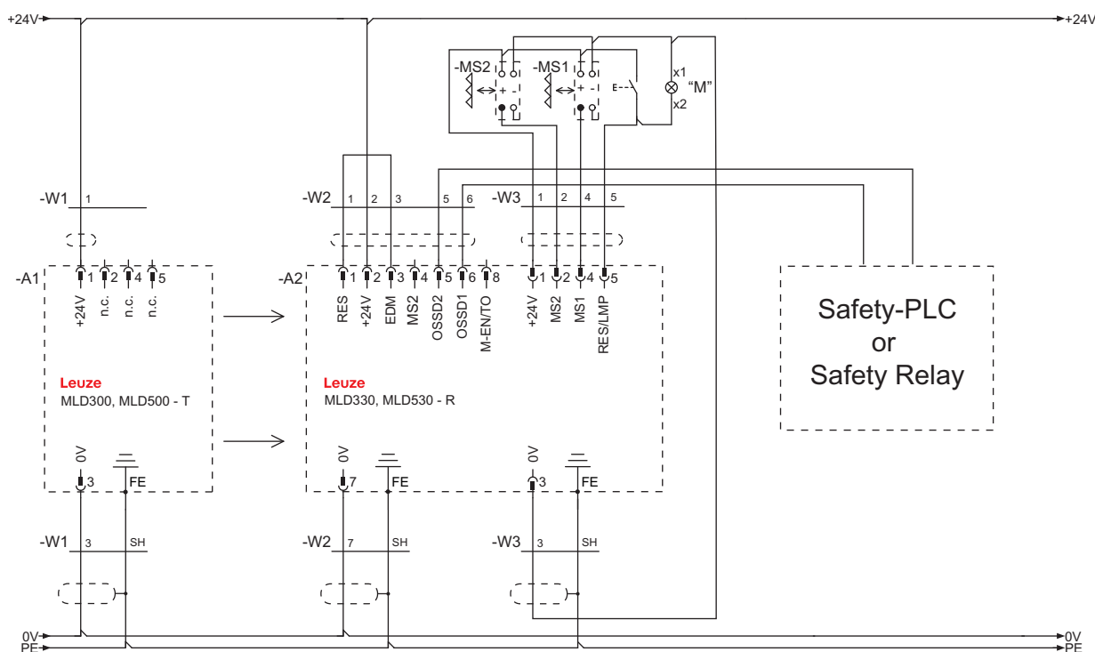
Fig. 7.16: Ejemplo de conexión MLD 330, MLD 530 (sistema emisor-receptor): muting de 2 sensores con control secuencial con timeout de muting 100 h (conexión transceptor analógico al respecto)
