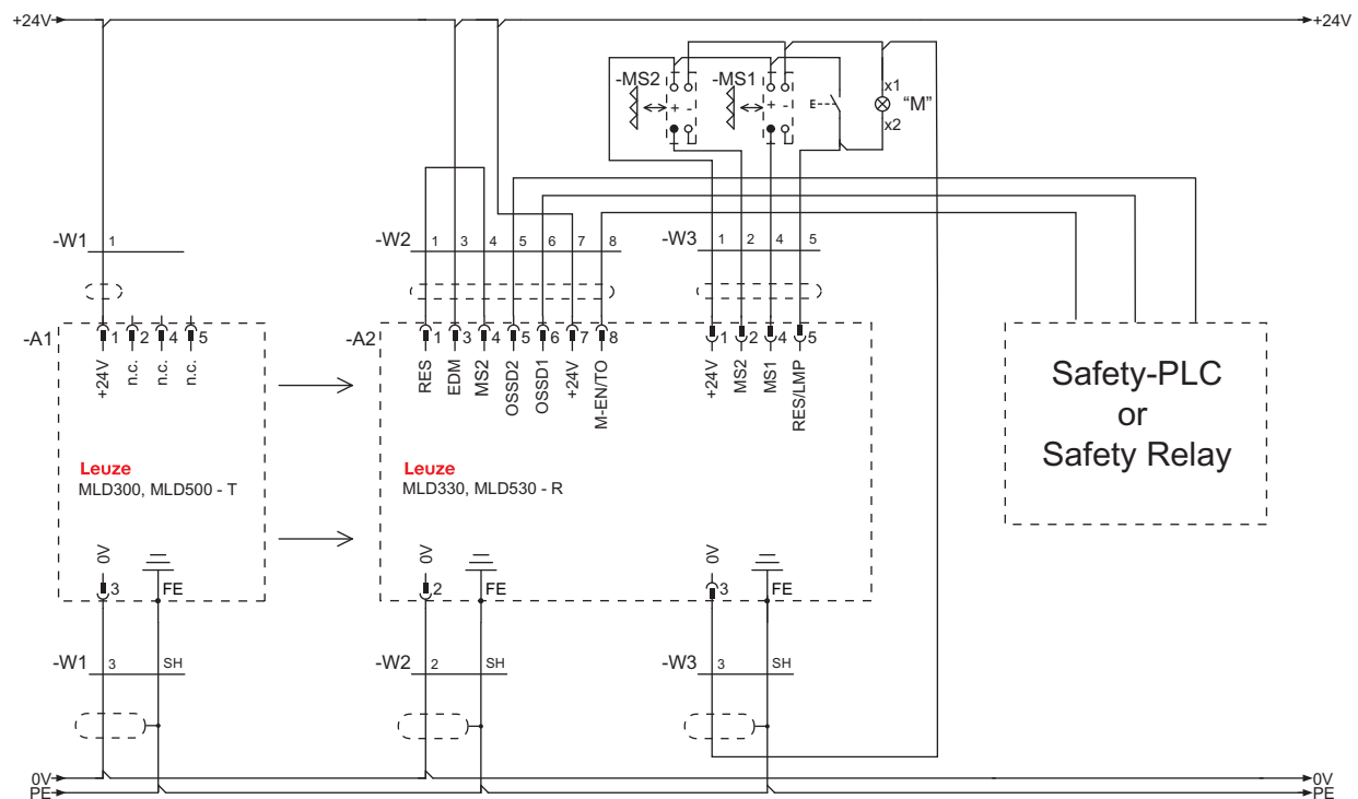
Fig. 7.17: Ejemplo de conexión MLD 330, MLD 530 (sistema emisor-receptor): Muting-Enable (conexión transceptor analógico al respecto)
