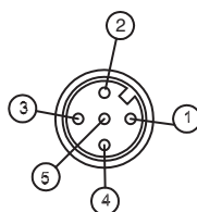
Fig. 7.6: Asignación de conector del MLD 500/AS-i (emisor, receptor/transceptor, conector hembra para lámpara de muting externa)
