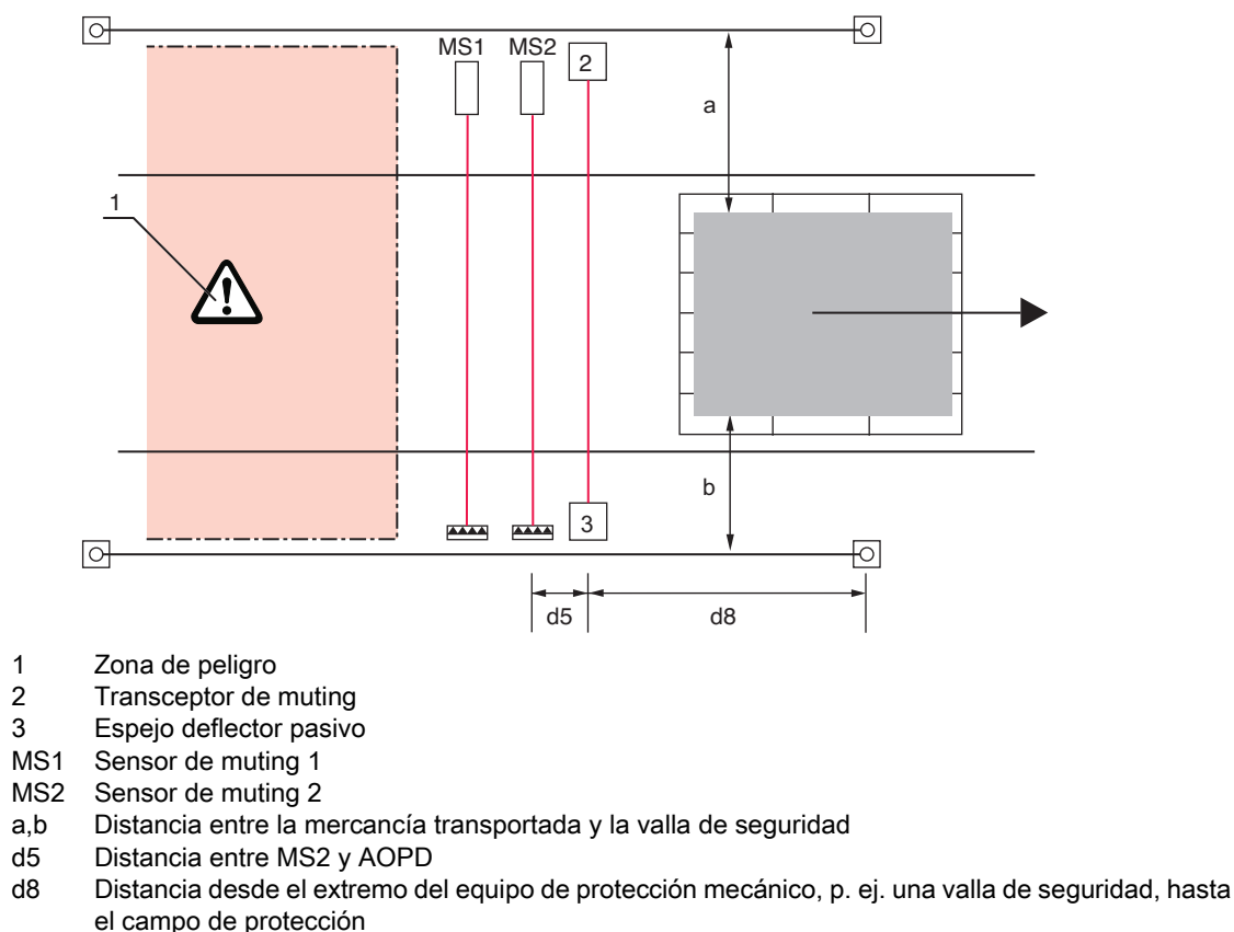
Fig. 6.10: Disposición típica de los sensores de muting en el muting de 2 sensores con control secuencial (ejemplo según IEC 62046)
