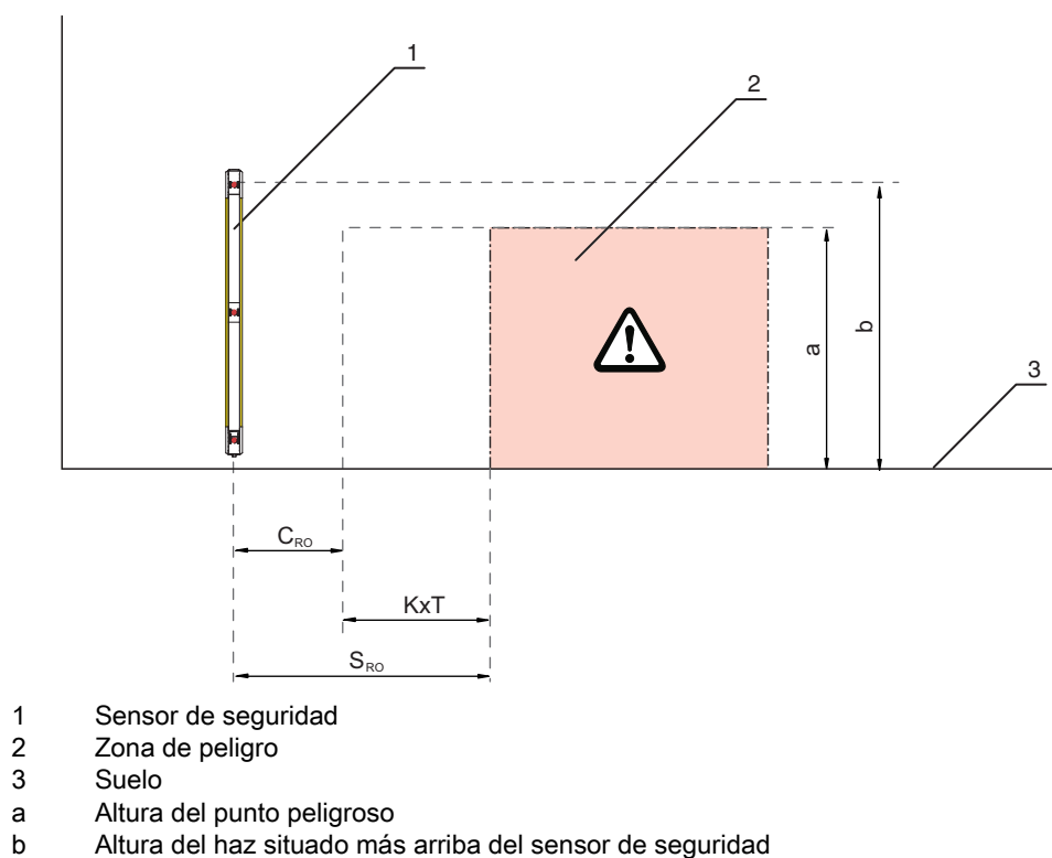
Fig. 6.2: Suplemento a la distancia de seguridad en caso de acceso por arriba o por abajo
