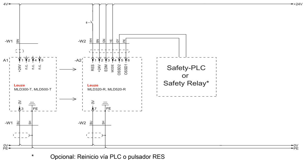
Fig. 7.7: Ejemplo de conexión MLD 320, MLD 520 (sistema emisor-receptor) sin EDM, con RES (conexión transceptor analógico al respecto)
