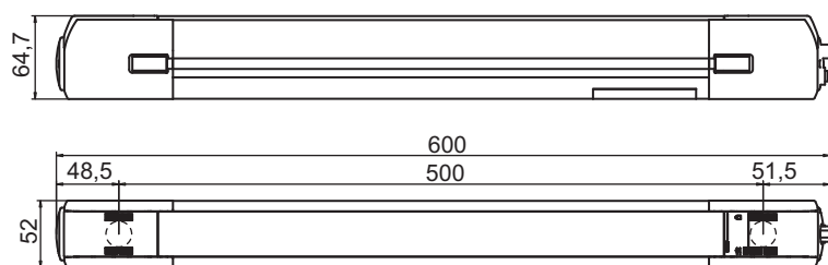
Fig. 14.2: Medidas MLD, emisor de 2 haces, receptor
