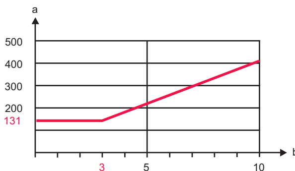
Fig. 6.3: Distancia mínima respecto a las superficies reflectantes según la anchura del campo de protección
