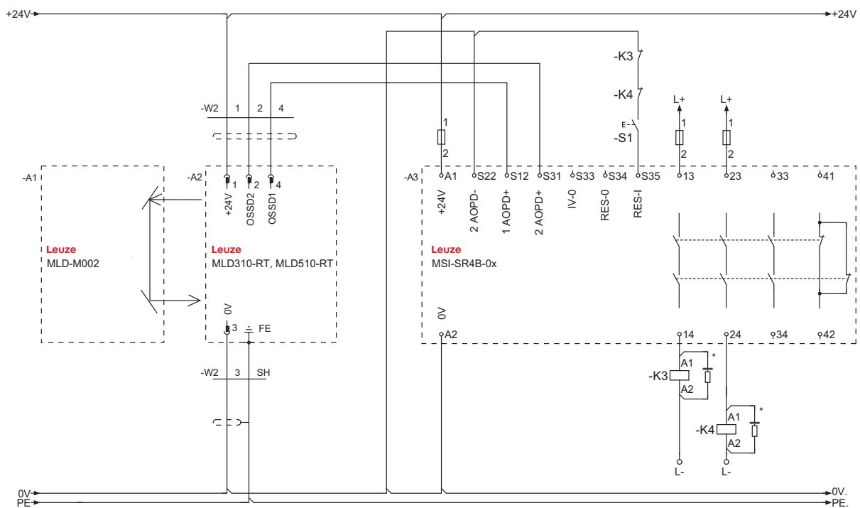
Fig. 7.8: Ejemplo de conexión MLD 510 (sistema transceptor) con EDM; RES en el micro de seguridad sin enclavamiento MSI-SR4B-0x
