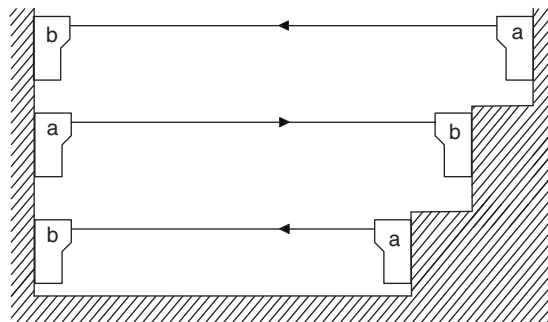
Fig. 6.1: Disposición multiaxial con asimetría geométrica (máx. 15 m)
