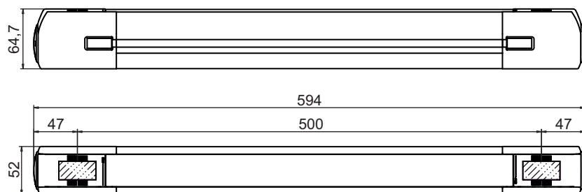
Fig. 14.7: Medidas MLD-M, espejo deflector de 2 haces
