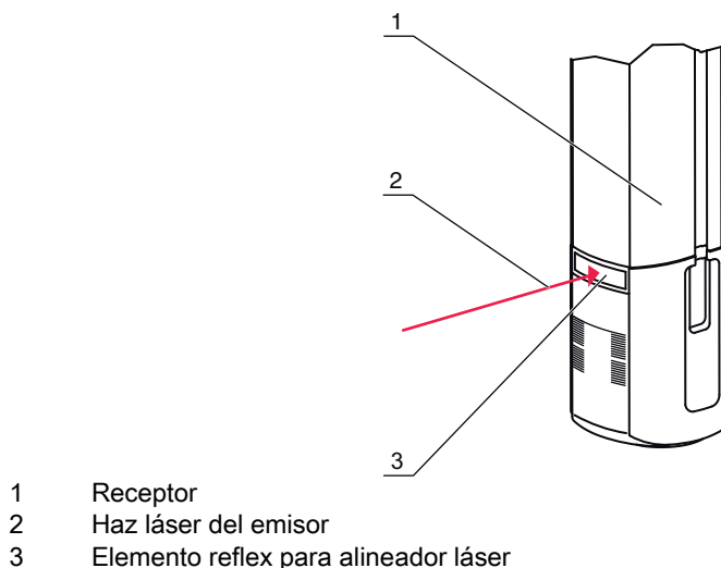
Fig. 8.3: Aplicar un alineador láser integrado: el haz láser del emisor alcanza el elemento reflex en el receptor y lo lleva a relucir de tal forma que sea visible desde lejos
