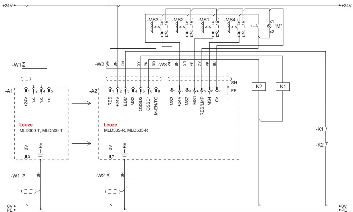
Fig. 7.14: Ejemplo de conexión MLD 335, MLD 535 (sistema emisor-receptor): muting de 4 sensores con control temporizado (conexión transceptor analógico al respecto)
