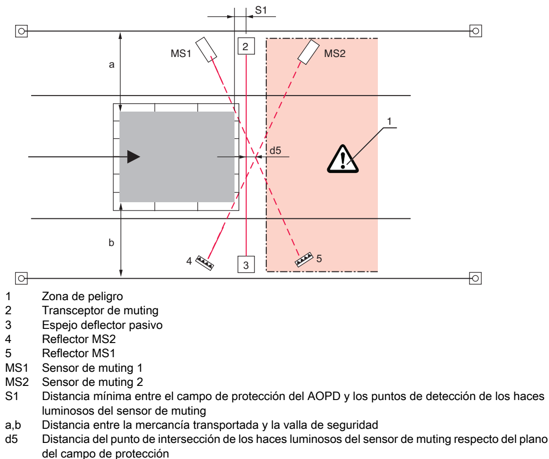
Fig. 6.8: Disposición típica de los sensores de muting en el muting de 2 sensores con control temporizado (ejemplo según IEC 62046)
