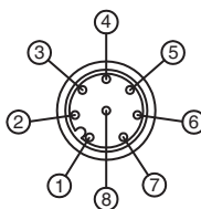
Fig. 7.4: Asignación de la hembrilla de 5 polos de los receptores MLD 330, MLD 530
