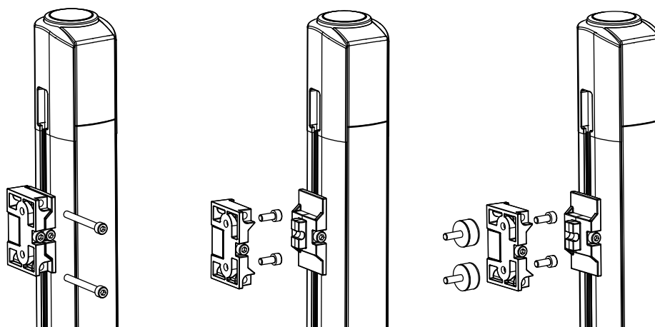
Fig. 6.16: Soporte orientable de sujeción BT-2SB10
