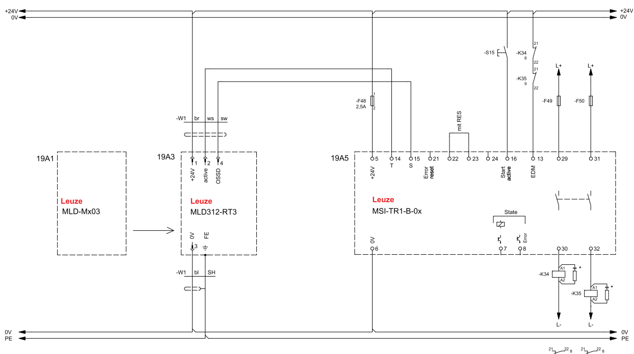
Fig. 7.10: Ejemplo de conexión MLD 312 (sistema emisor-receptor) y MSI-TR1B-0x, con EDM y RES
