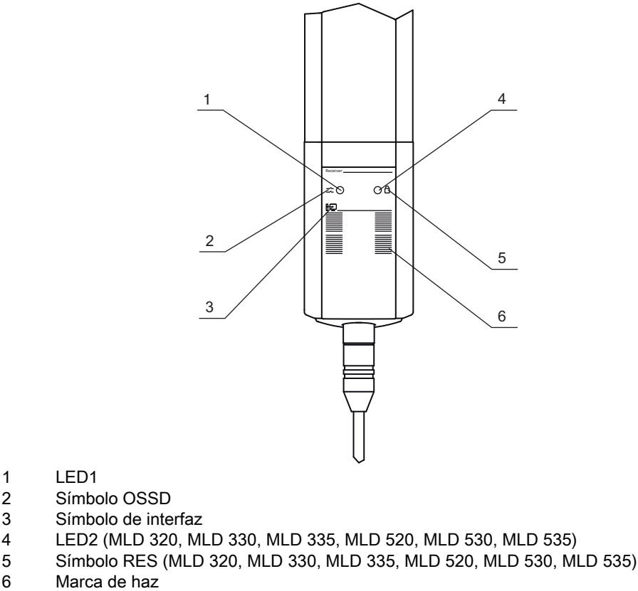
Fig. 3.4: Indicadores de funcionamiento en el receptor
