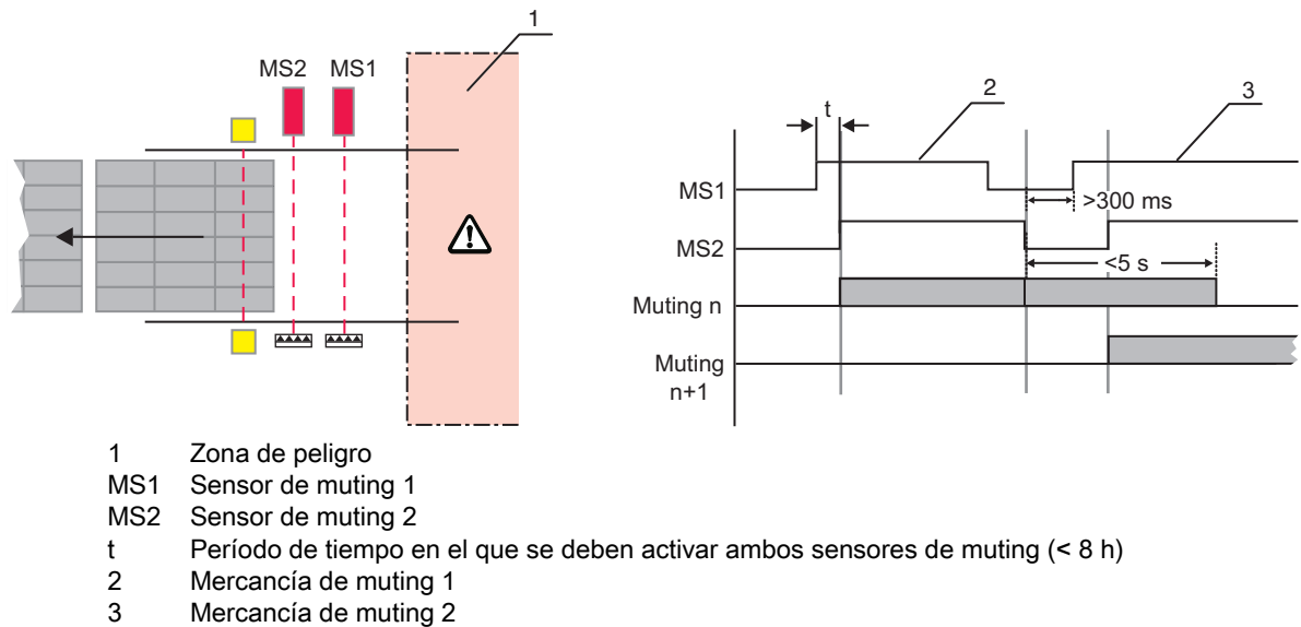
Fig. 4.4: Muting en caso de sucesión de objetos compacta: disposición de los sensores de muting y terminación del tiempo
