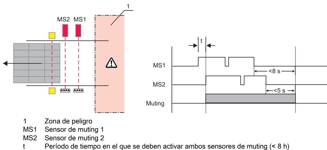
Fig. 4.3: Muting de 2 sensores con control secuencial - disposición de los sensores de muting y terminación del tiempo
