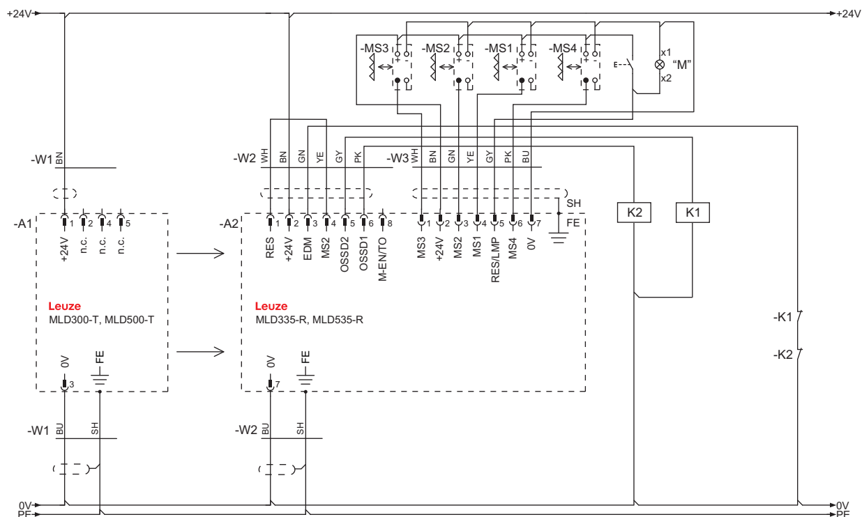
Fig. 7.12: Ejemplo de conexión MLD 335, MLD 535 (sistema emisor-receptor): muting de 4 sensores con control temporizado con timeout de muting 10 min (conexión transceptor analógico al respecto)
