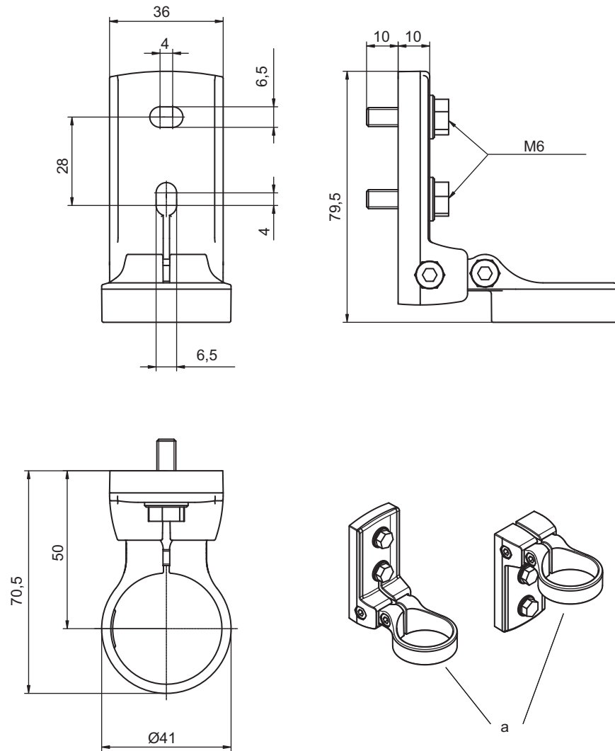
Fig. 14.10: Soporte giratorio BT-240C
