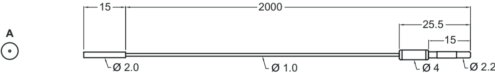
A Núcleo de fibra de plástico Ø 0,25 mm x 1 ud.
