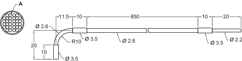
A Ø 0.265 mm 玻璃纤维芯 x 32 件
