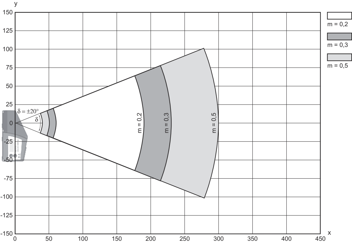
Curva del campo di lettura laterale
