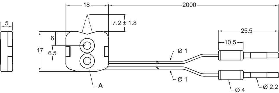
A 2 x Ø 3,2 / Ø 6,2 (orificio de montaje, en el lado frontal)
