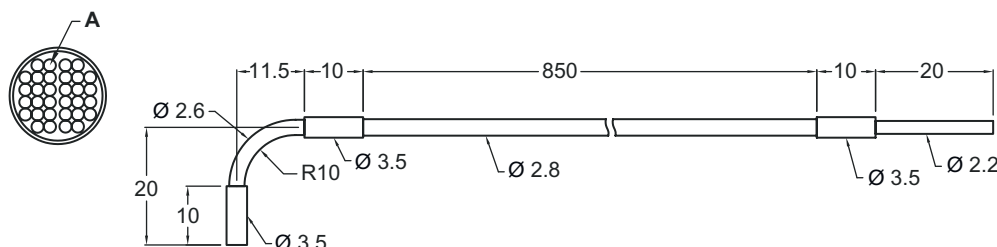
A Noyau de fibres plastiques Ø 0,265 mm x 32 unités
