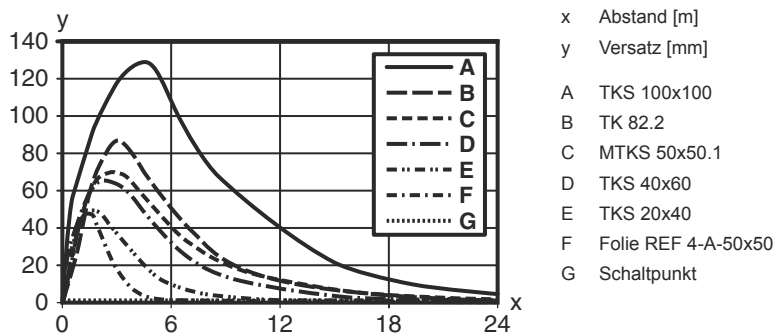
Typ. Funktionsreserve
