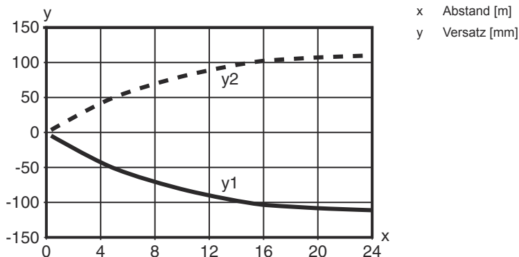
Typ. Ansprechverhalten (TKS100x100)
