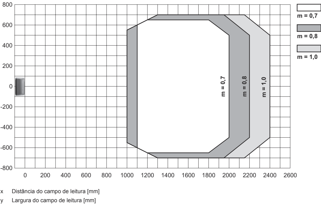
Curva do campo de leitura
