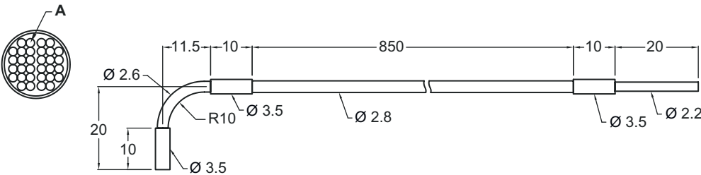
A Núcleo de fibra de plástico Ø 0,265 mm x 32 uds.
