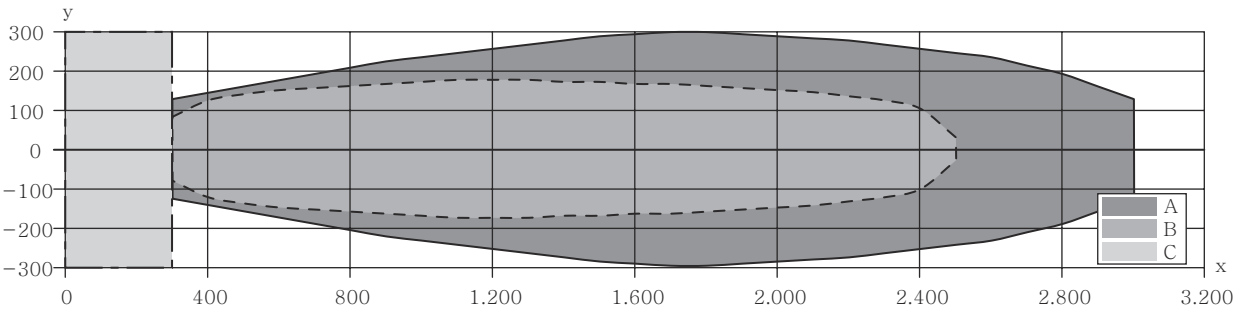
Typ. Ansprechverhalten
