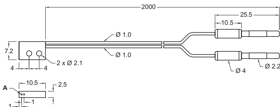
A Noyau de fibres plastiques Ø 0,5 mm x 2 unités
